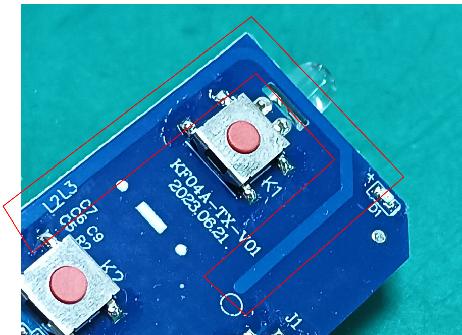
Antenna
