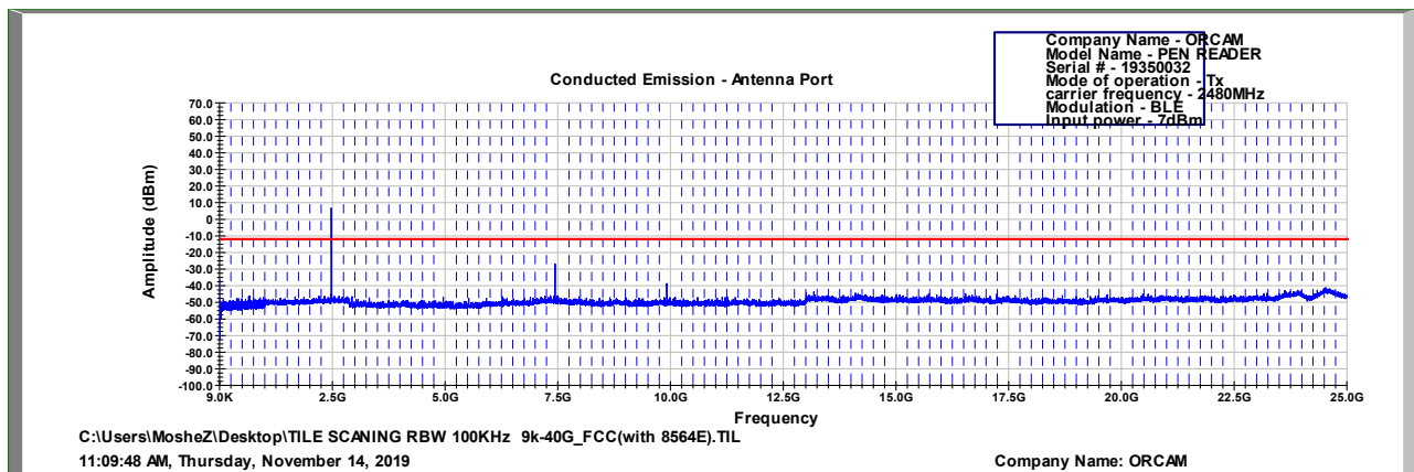
Figure 98 2480.0 MHz, BLE
