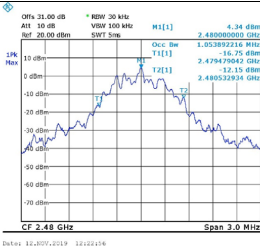
Figure 84. 2480.0 MHz, BLE
