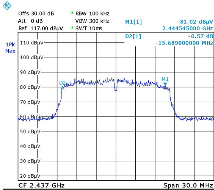
Figure 24. 2437.0MHz - Wi-Fi/g
