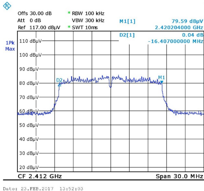
Figure 23. 2412.0MHz - Wi-Fi/g
