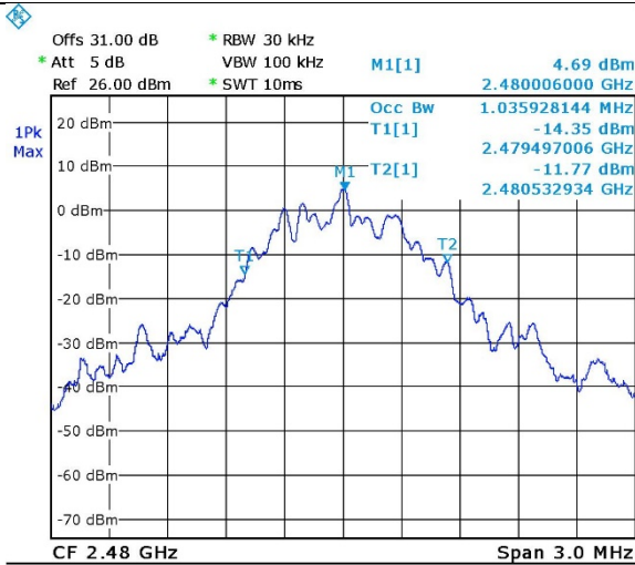
Figure 84. 2480.0 MHz, BLE
