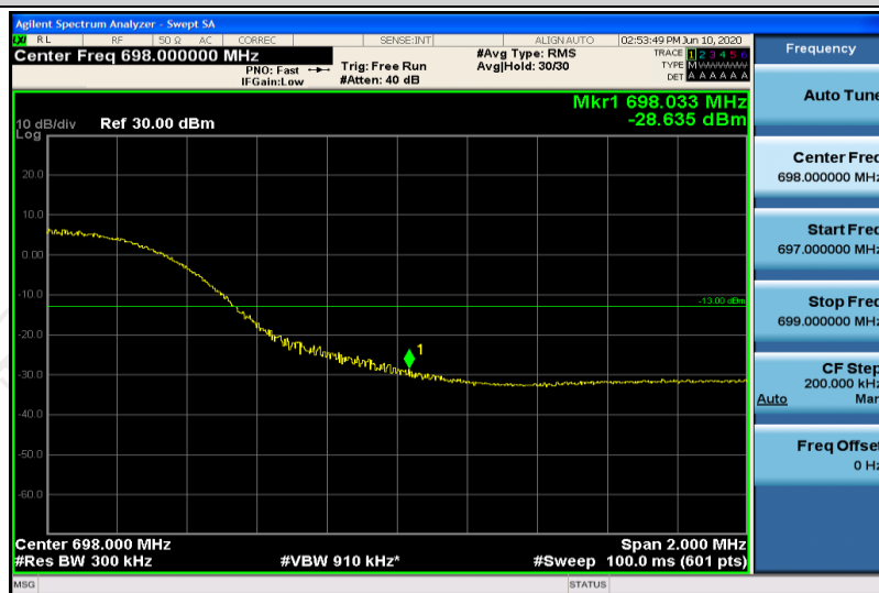
Band71-20MHz-QPSK-133222-1RB#99
