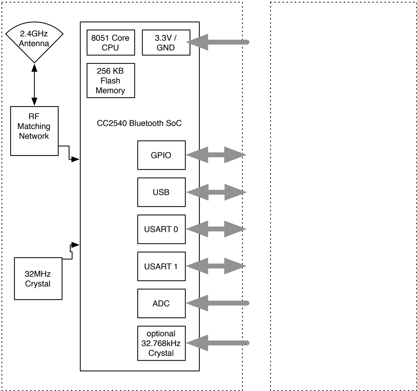
LBM313-2540-256 Module
