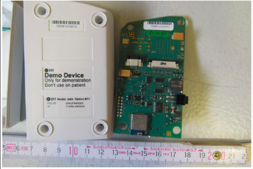
PCB bottom
