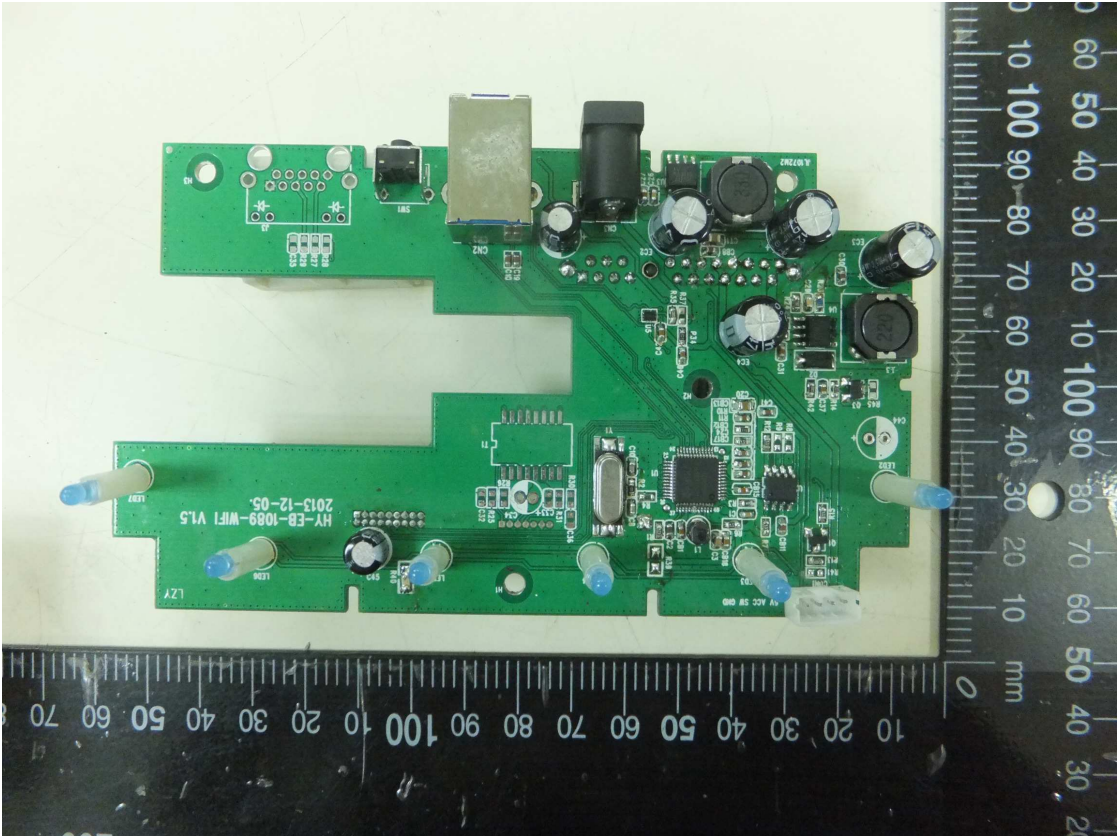
05 PCB1-F
