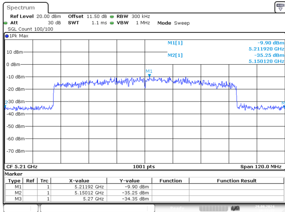
-26dB Bandwidth NVNT ax80 5210MHz Ant1
