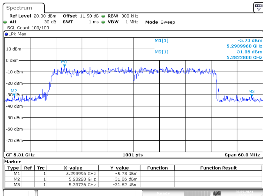
-26dB Bandwidth NVNT ax40 5310MHz Ant1
