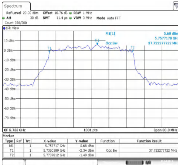
11AX40MIMO-Ant1-5755
