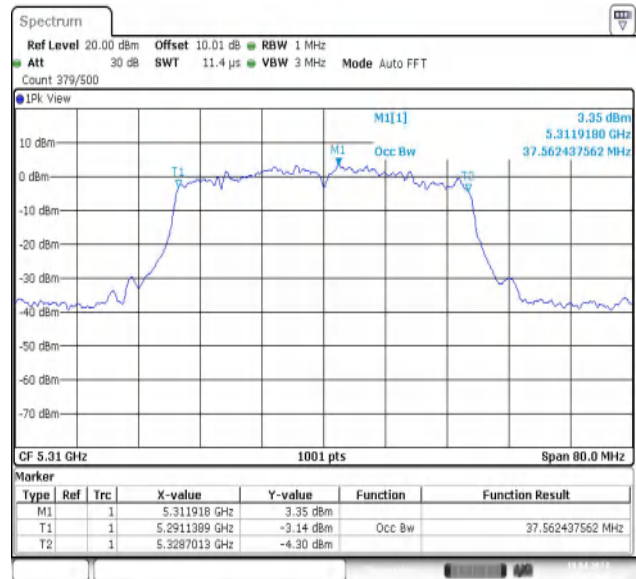
11AX40MIMO-Ant2-5310
