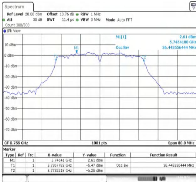
11AC40MIMO-Ant1-5755
