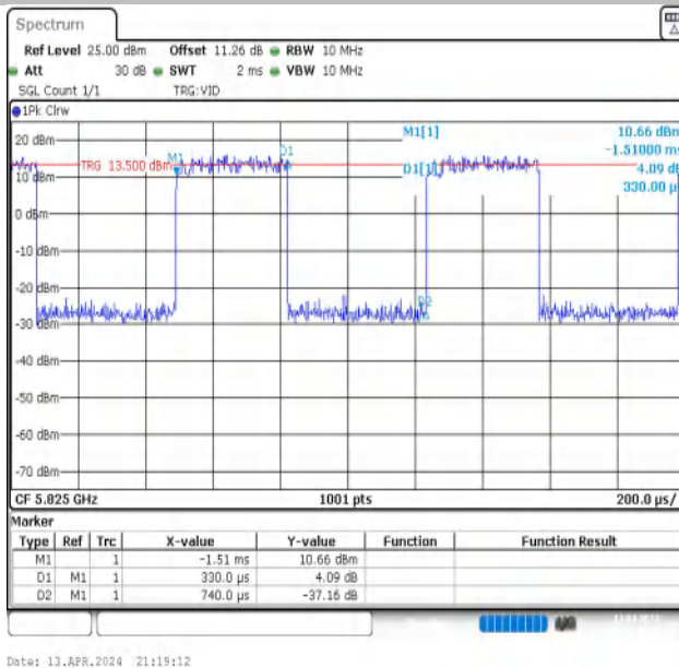
NTNV-11N20MIMO-Ant1-5825
