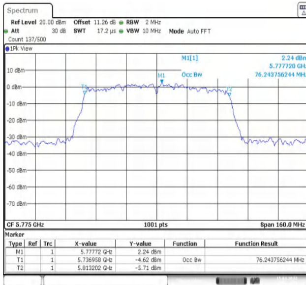
11AC80MIMO-Ant1-5775
