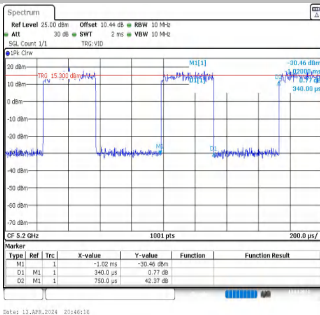
NTNV-11N20MIMO-Ant1-5200
