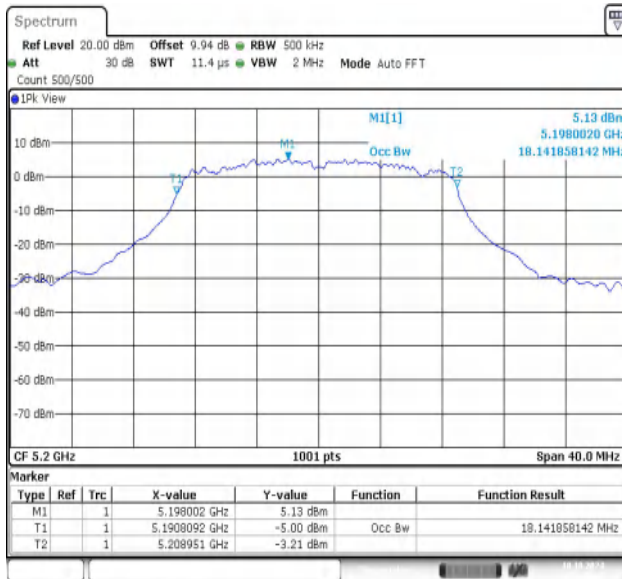
11AC20MIMO-Ant1-5200
