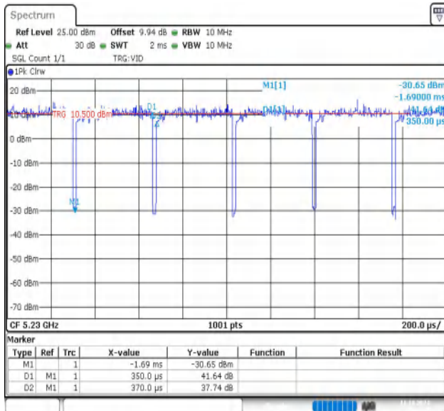
NTNV-11AC40MIMO-Ant1-5230
