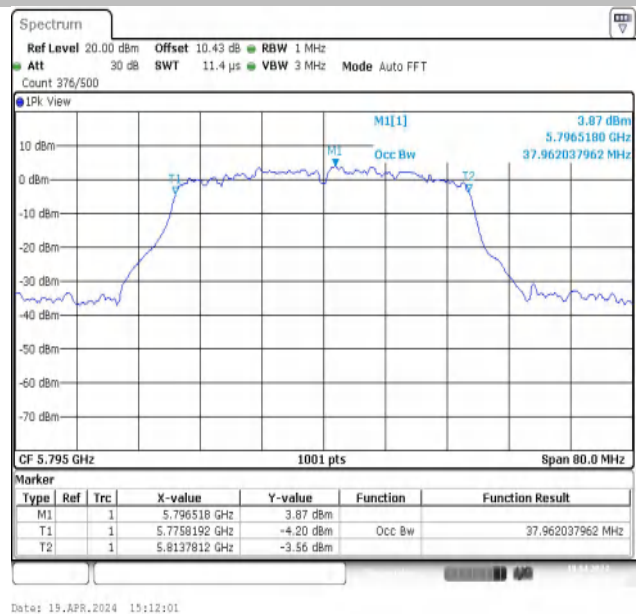
11AX40MIMO-Ant2-5795
