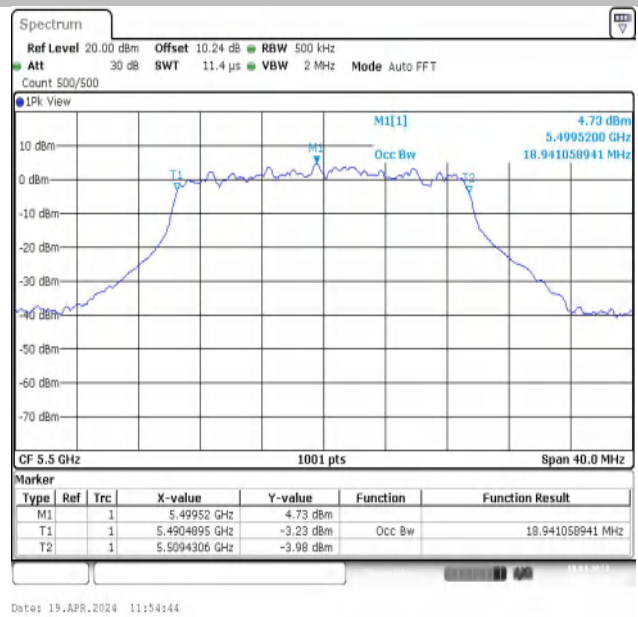
11AX20MIMO-Ant2-5500
