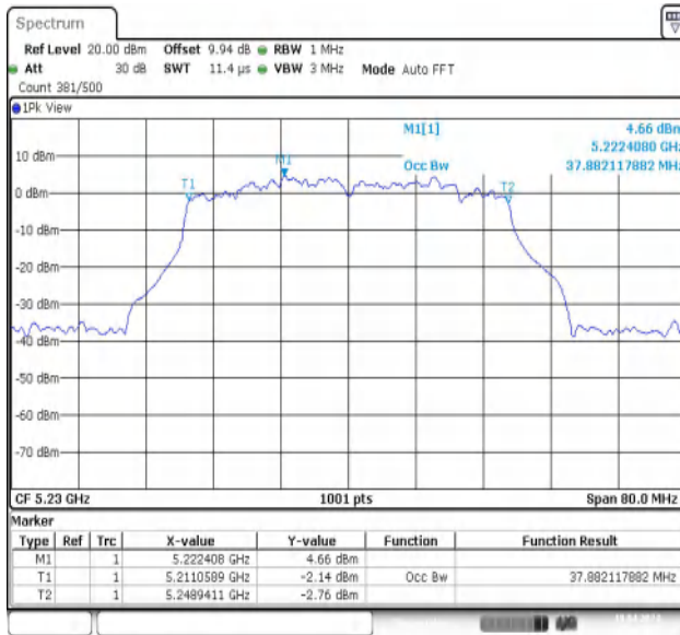
11AX40MIMO-Ant1-5230
