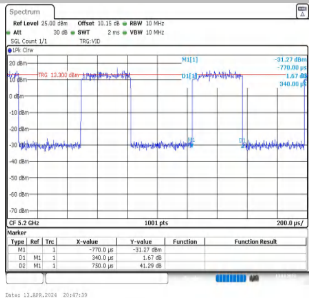
NTNV-11N20MIMO-Ant2-5200
