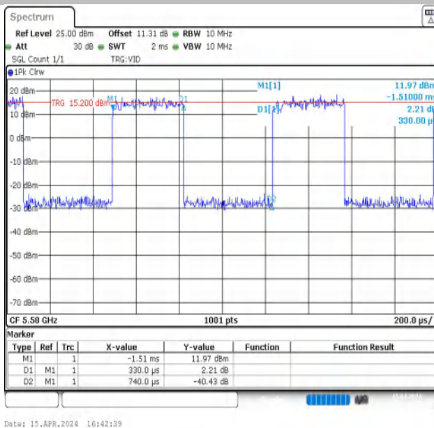
NTNV-11N20MIMO-Ant1-5580
