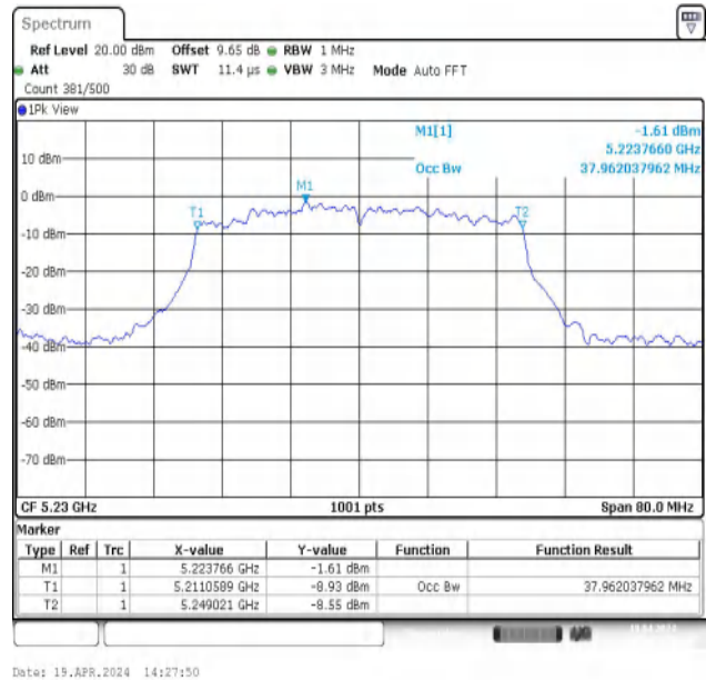
11AX40MIMO-Ant2-5230
