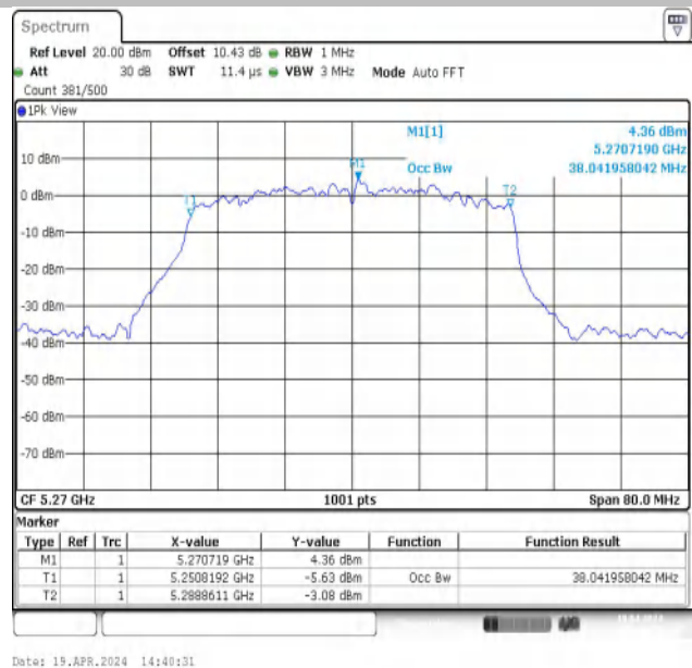
11AX40MIMO-Ant2-5270
