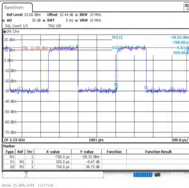
NTNV-11N40MIMO-Ant1-5230
