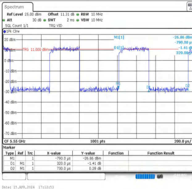
NTNV-11N40MIMO-Ant1-5550
