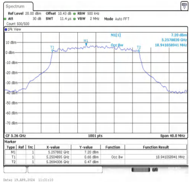
11AX20MIMO-Ant2-5260
