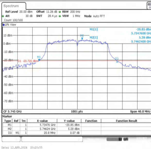
11A-Ant1-5745
