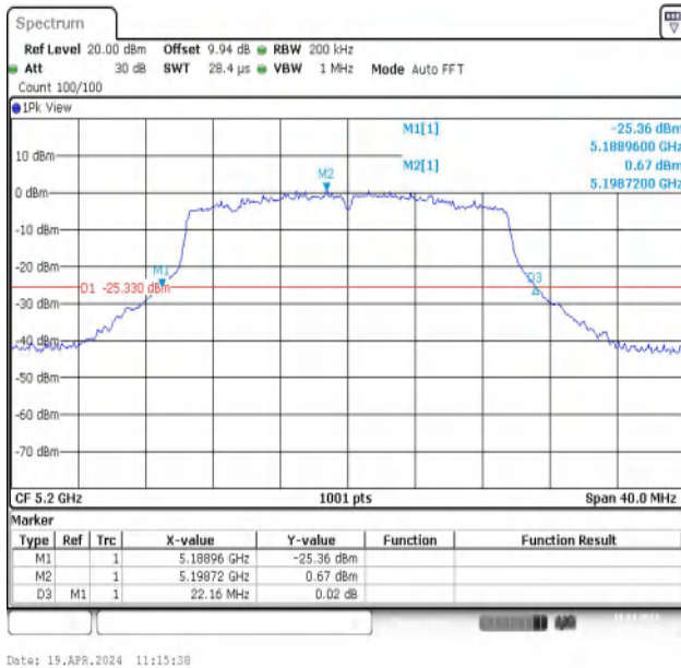
11AX20MIMO-Ant1-5200
