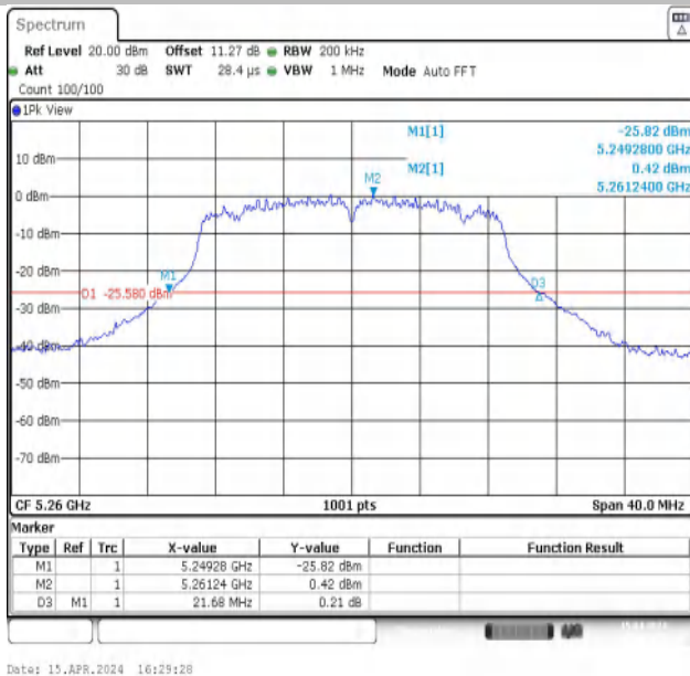
11N20MIMO-Ant1-5260
