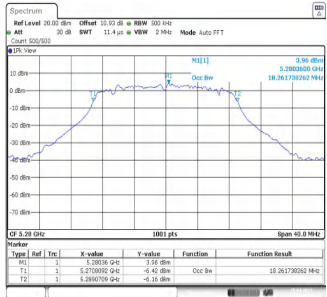
11N20MIMO-Ant2-5280
