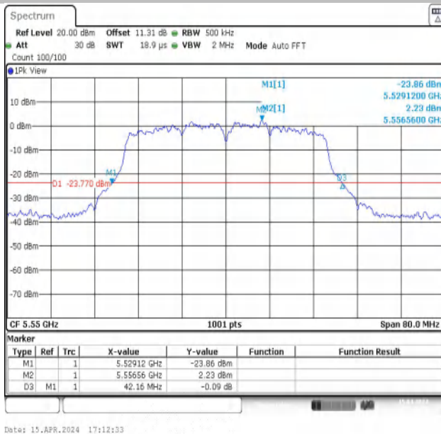
11N40MIMO-Ant1-5550
