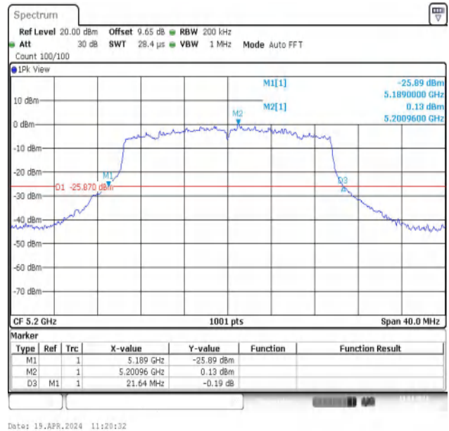
11AX20MIMO-Ant2-5200
