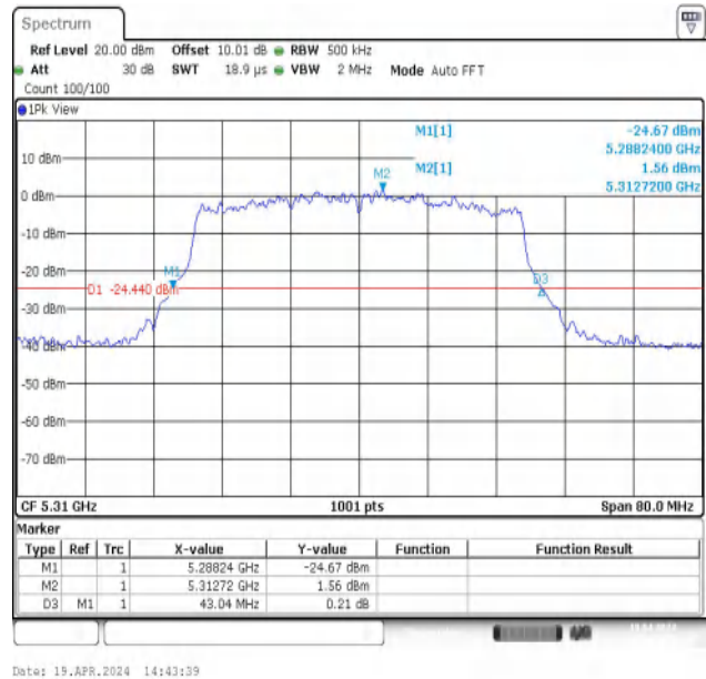
11AX40MIMO-Ant2-5310
