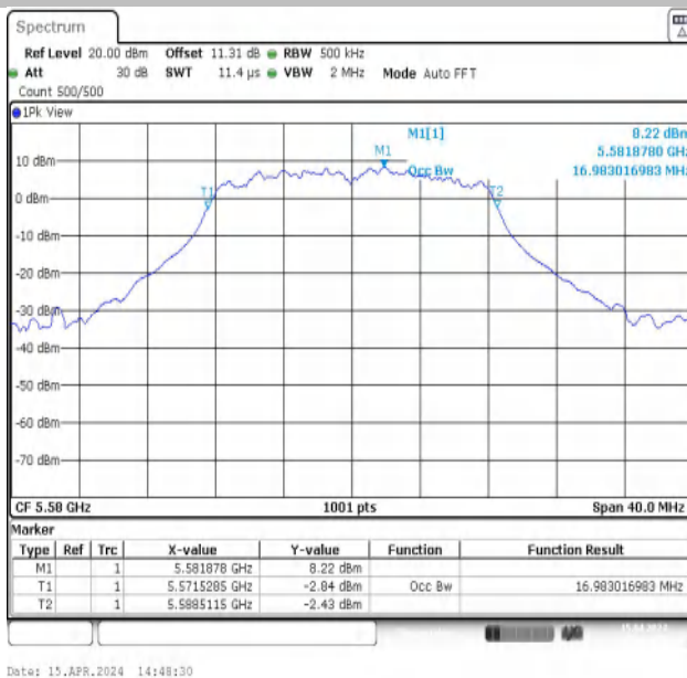
11A-Ant1-5580
