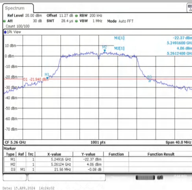
11A-Ant1-5260
