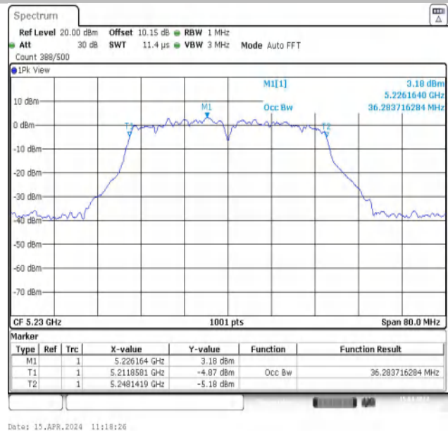
11N40MIMO-Ant2-5230
