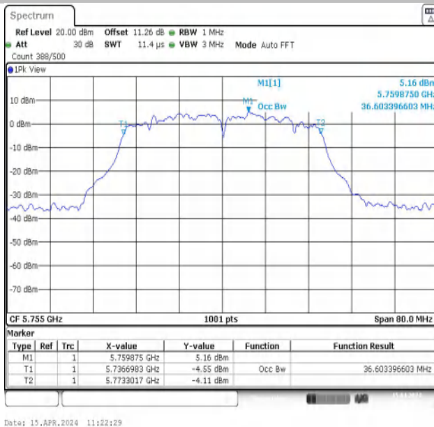
11N40MIMO-Ant1-5755
