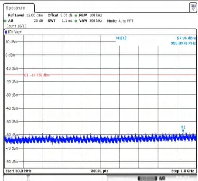
BLE_2M-Ant1-2440-30~1000-PASS
