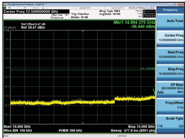
10 GHz – 15 GHz
