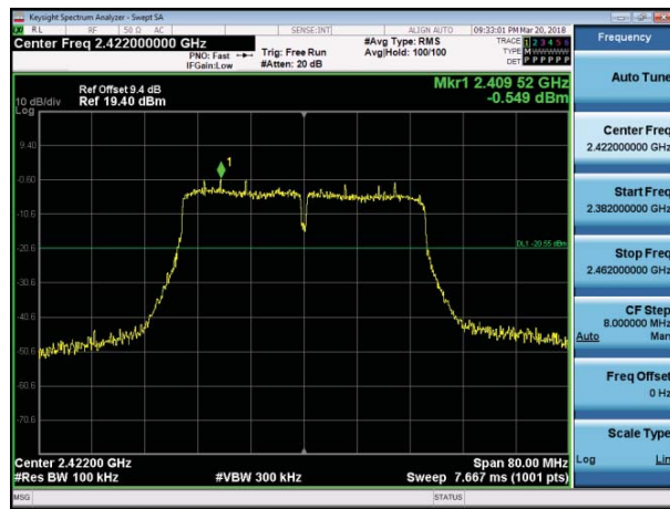
2382 MHz – 2462 MHz
