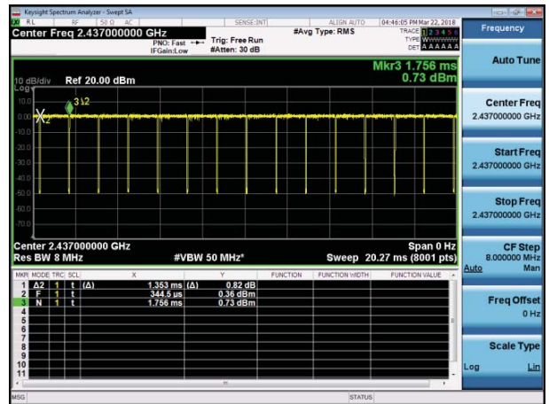
IEEE 802.11g
