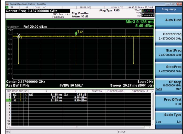
IEEE 802.11b
