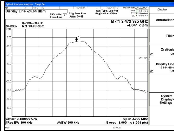
2477.5 MHz - 2482.5 MHz
