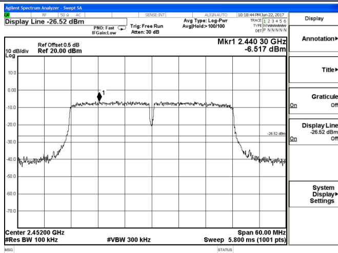
2422 MHz – 2482 MHz
