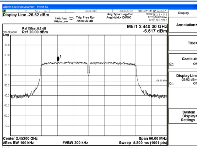
2422 MHz – 2482 MHz
