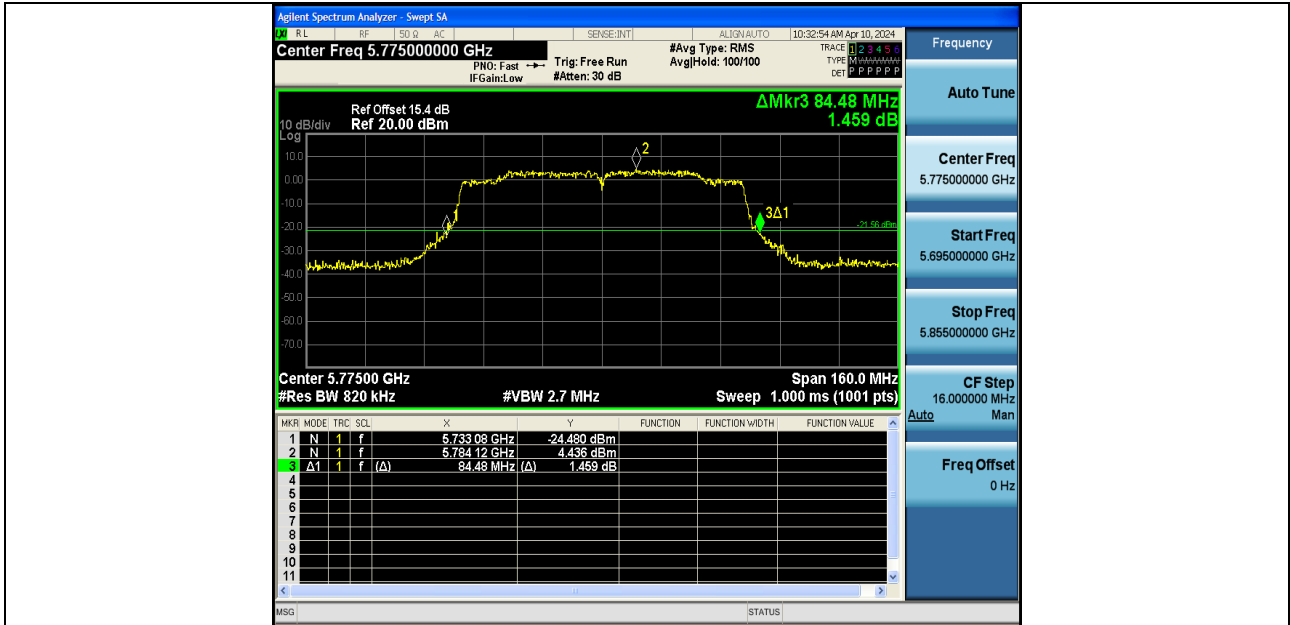
11AC80SISO-Ant1-5775
