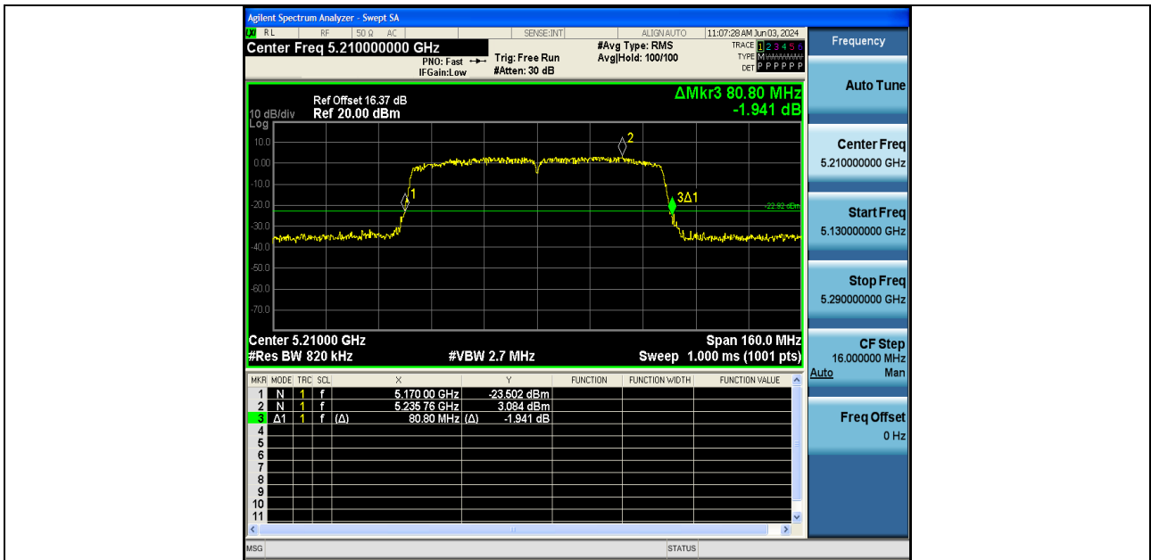
11AX80SISO-Ant2-5210
