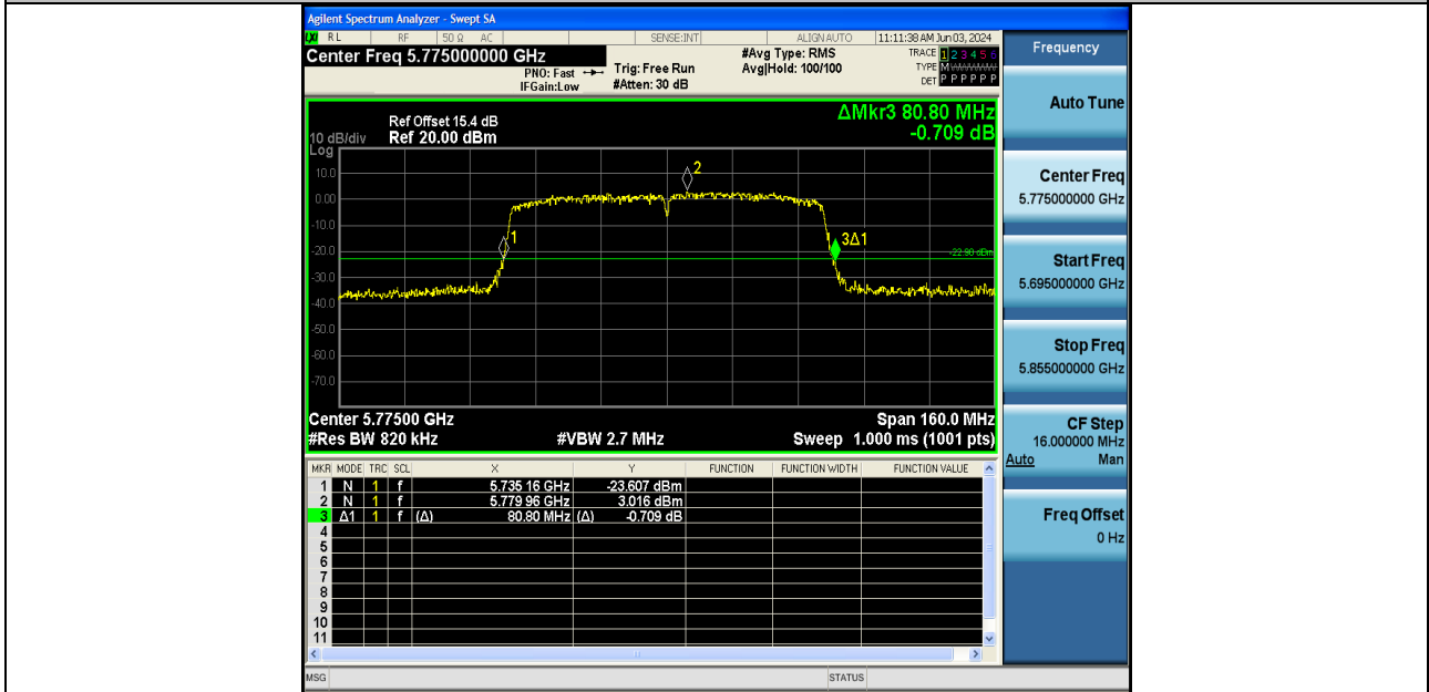
11AX80SISO-Ant2-5775
