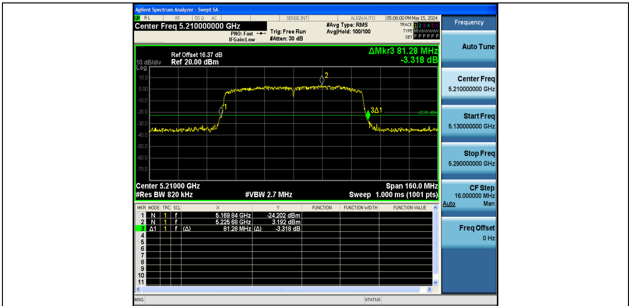
11AX80SISO-Ant1-5210
