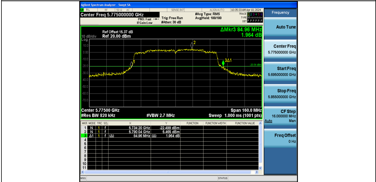
11AC80SISO-Ant2-5775
