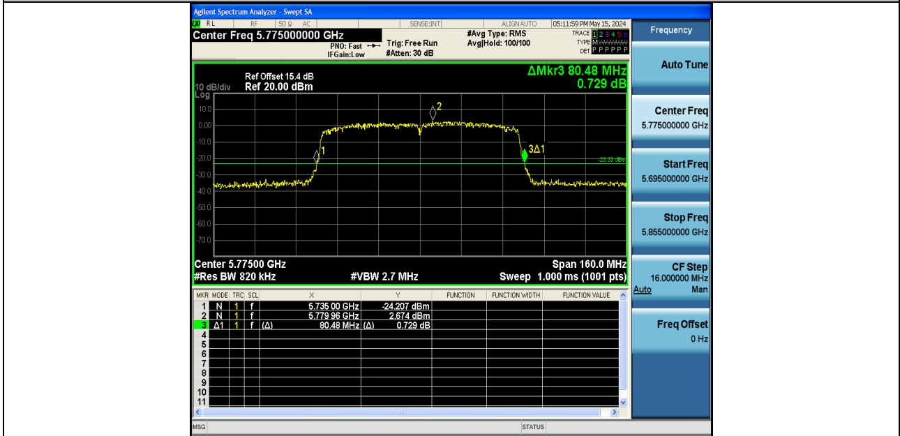
11AX80SISO-Ant1-5775
