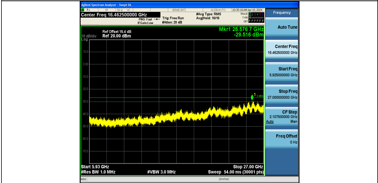
11AC80SISO-Ant1-5775-5925~27000-PASS
