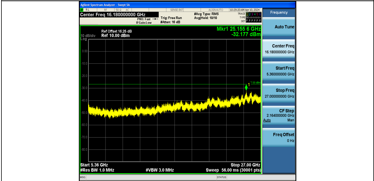
11AC80SISO-Ant2-5210-5360~27000-PASS
