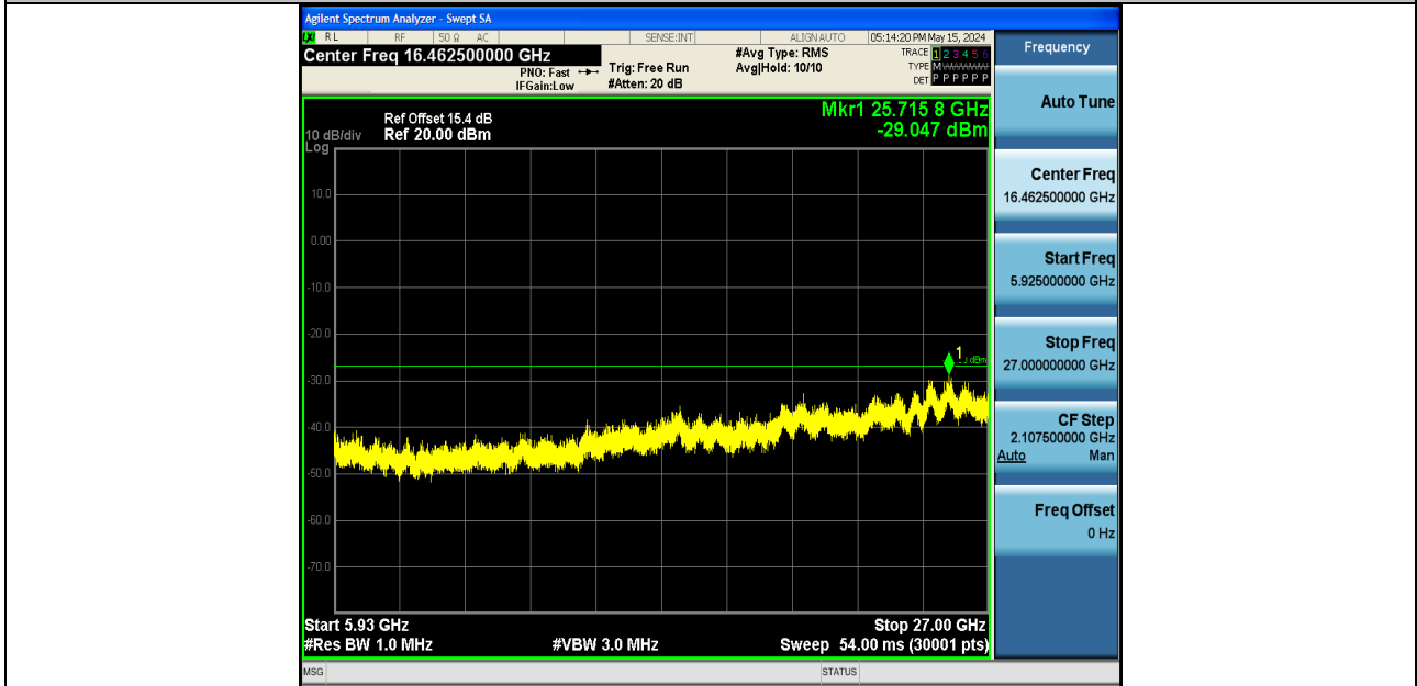
11AX80SISO-Ant1-5775-5925~27000-PASS
