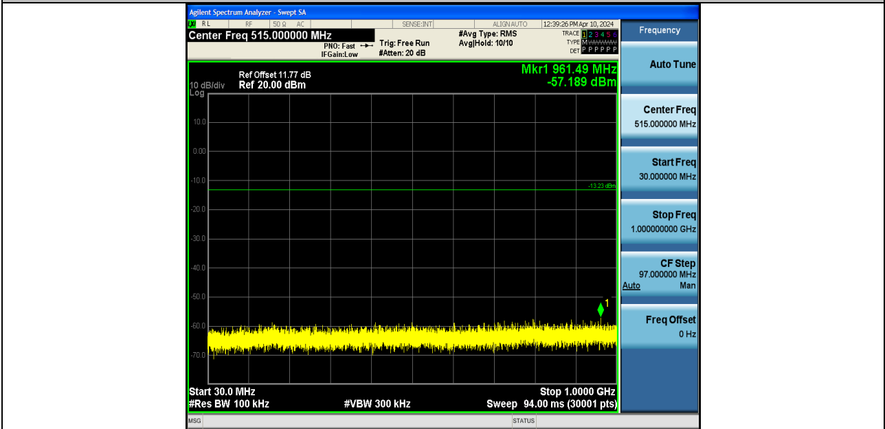
BLE_2M-Ant1-2440-30~1000-PASS
