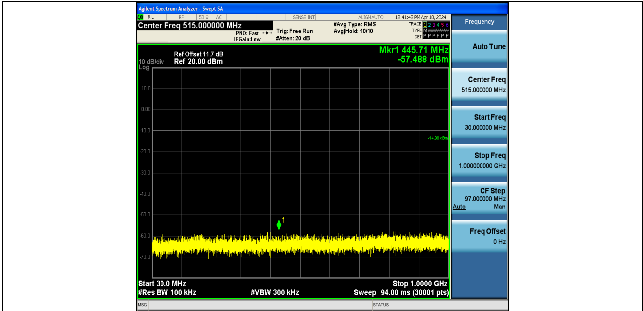
BLE_2M-Ant1-2480-30~1000-PASS
