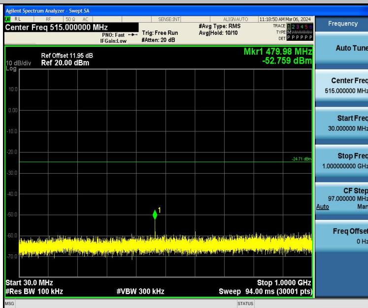
11G-Ant1-2412-30~1000-PASS
