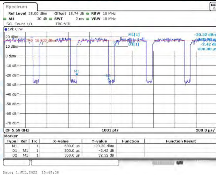
11AX80MIMO_Ant2_5690
