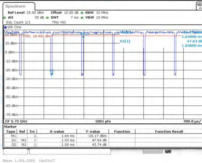
11AX20MIMO_Ant1_5720
