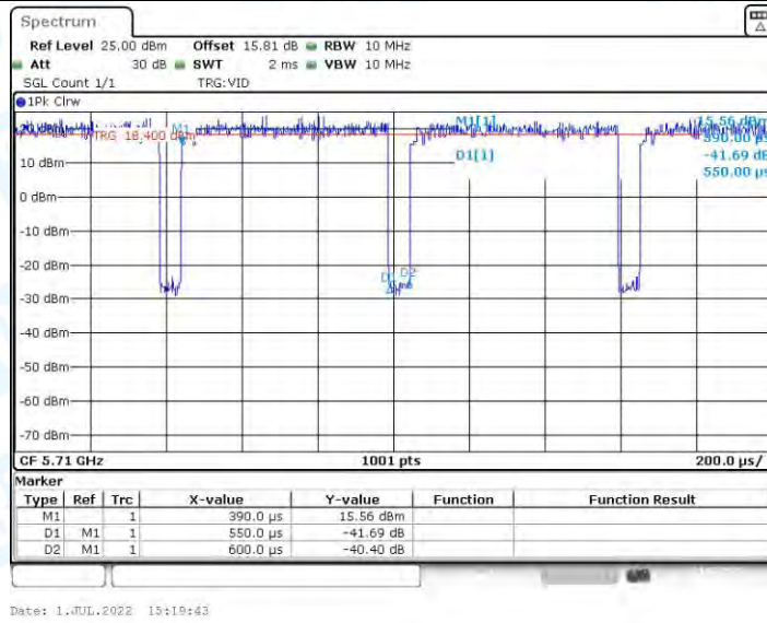
11AX40MIMO_Ant2_5710
