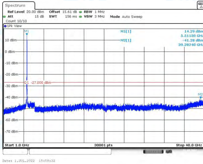
11AX40MIMO_Ant2_5510_1000~40000
