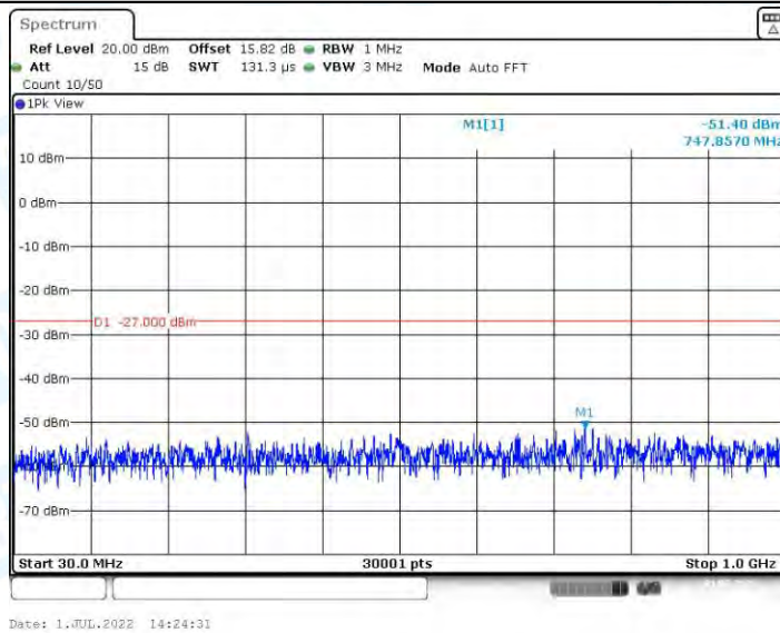
11AX20MIMO_Ant1_5720_30~1000
