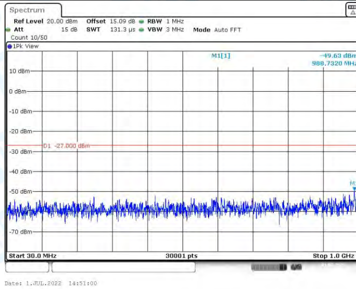
11AX40MIMO_Ant2_5190_30~1000
