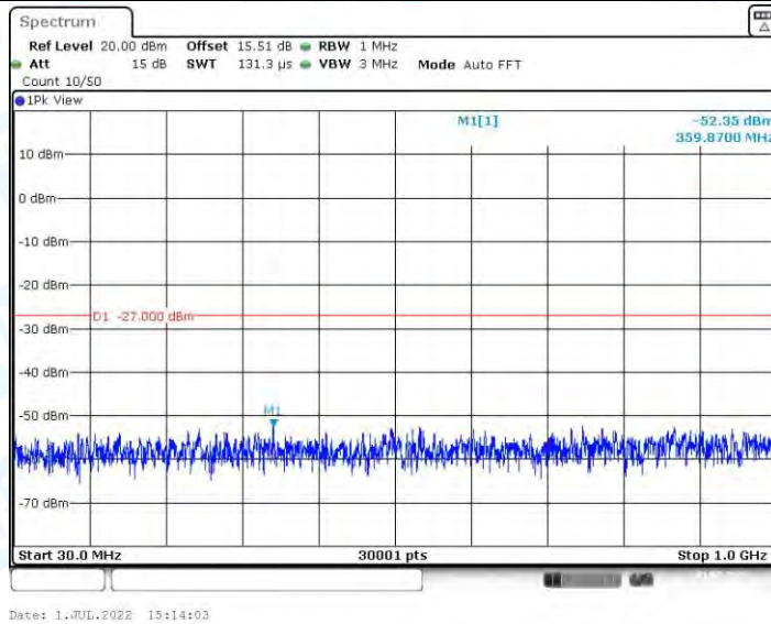
11AX40MIMO_Ant1_5550_30~1000
