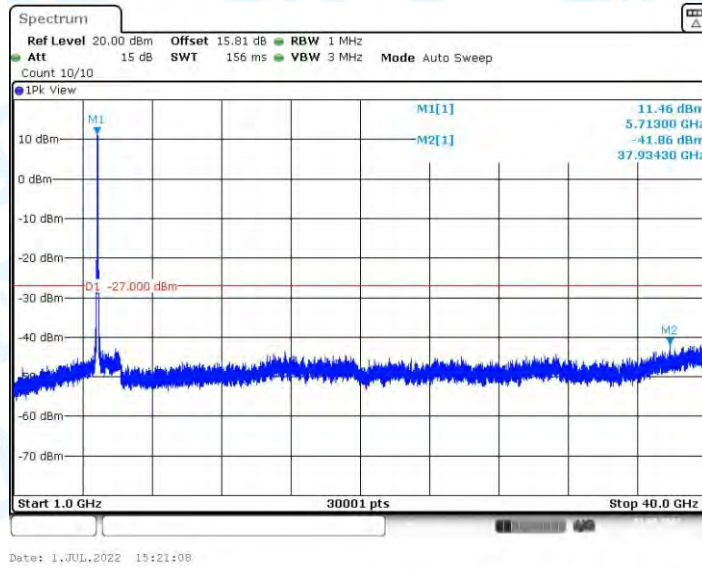
11AX40MIMO_Ant2_5710_1000~40000
