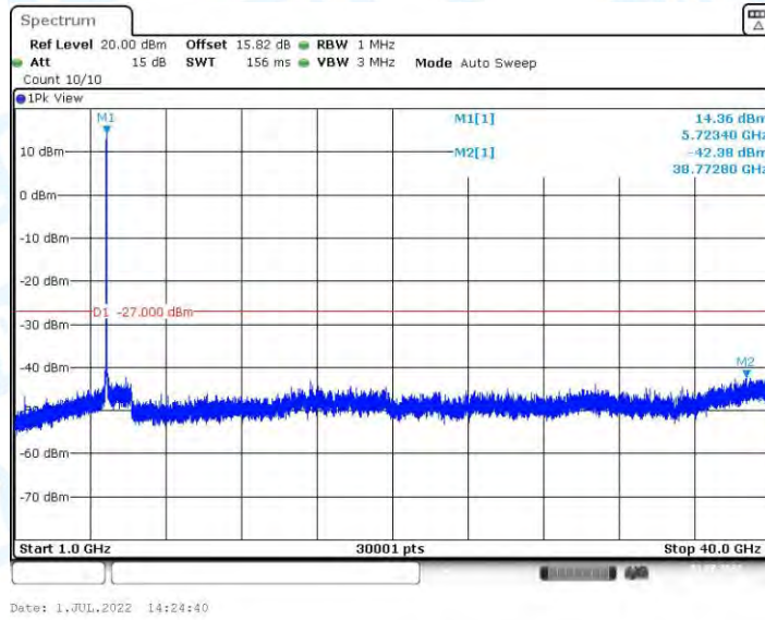
11AX20MIMO_Ant1_5720_1000~40000
