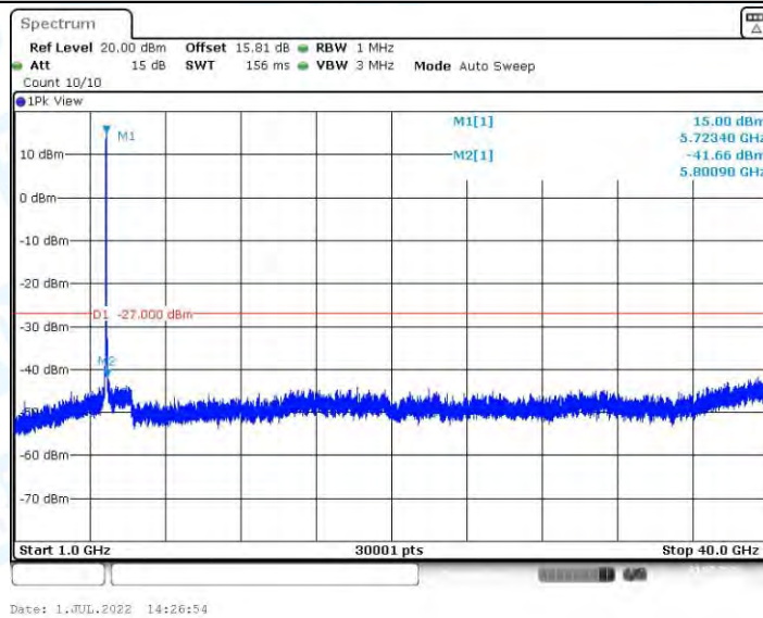
11AX20MIMO_Ant2_5720_1000~40000
