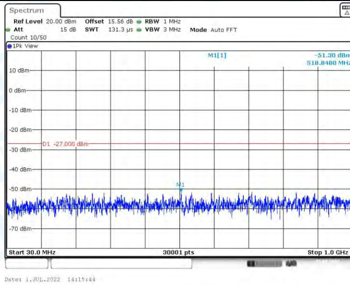
11AX20MIMO_Ant1_5500_30~1000
