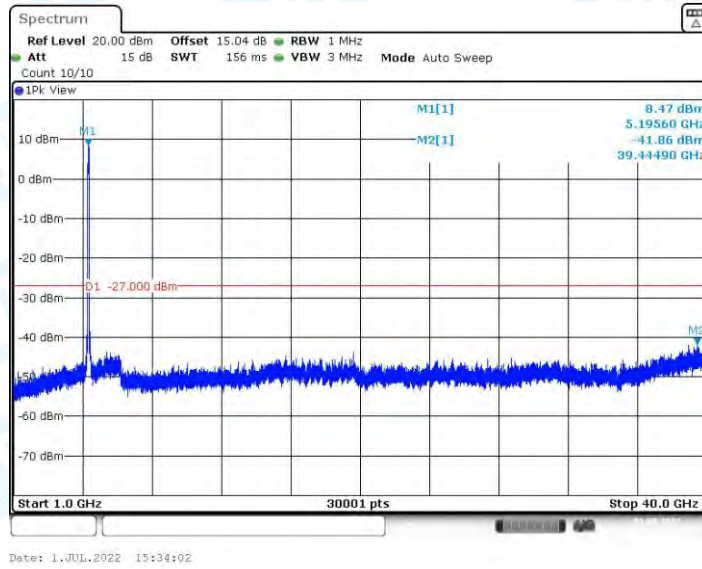
11AX80MIMO_Ant1_5210_1000~40000
