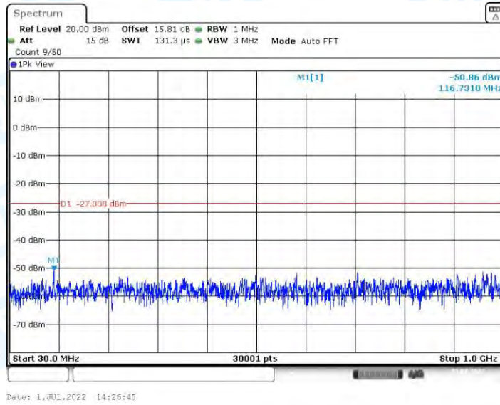
11AX20MIMO_Ant2_5720_30~1000
