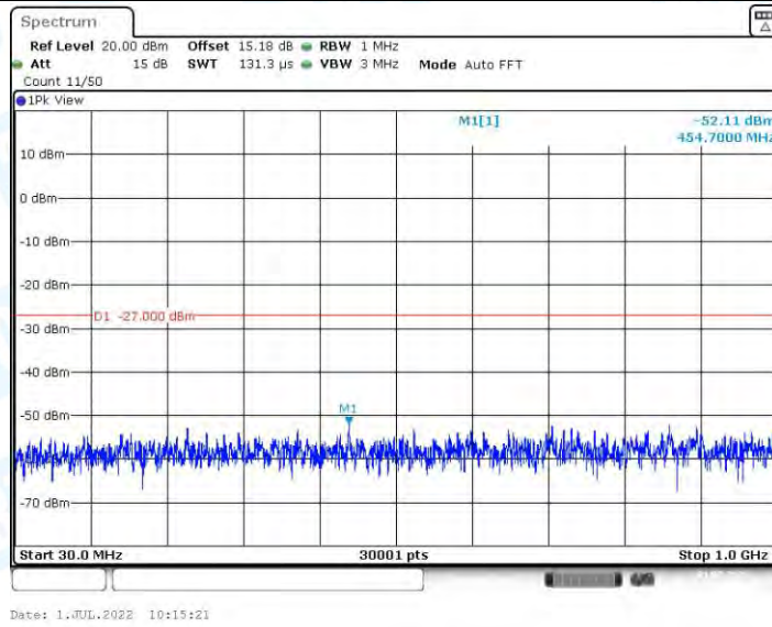
11AC40MIMO_Ant1_5230_30~1000
