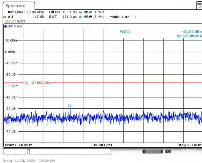
11AX40MIMO_Ant2_5710_30~1000
