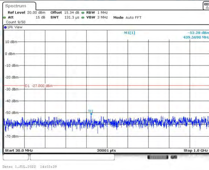
11AX20MIMO_Ant2_5260_30~1000
