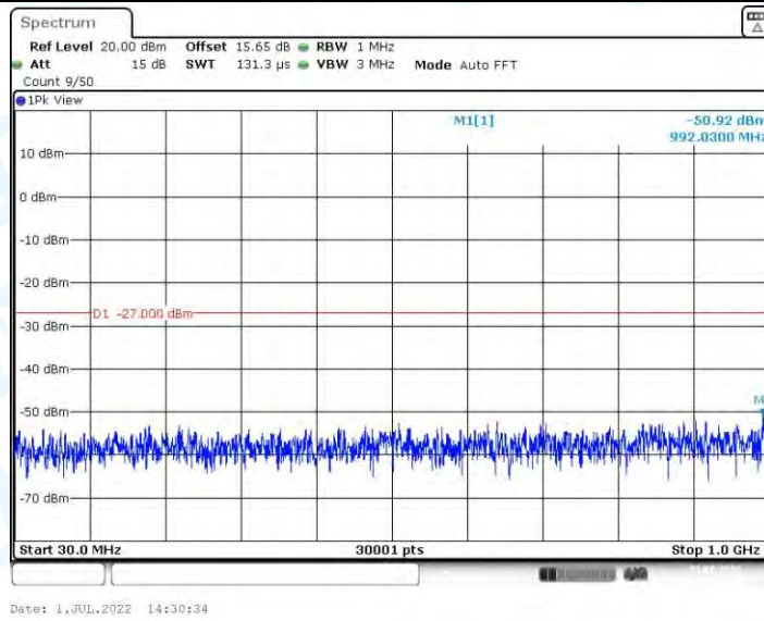
11AX20MIMO_Ant1_5745_30~1000
