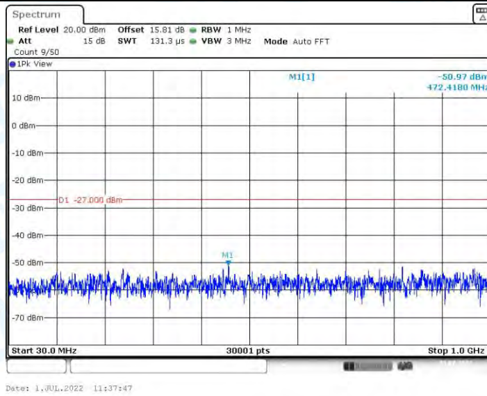
11AC40MIMO_Ant2_5710_30~1000
