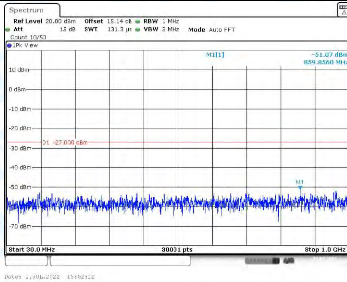
11AX40MIMO_Ant1_5310_30~1000
