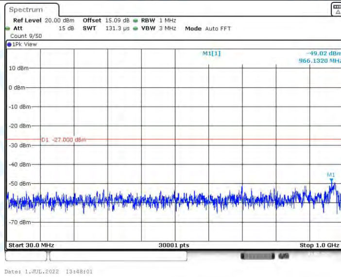
11AX20MIMO_Ant2_5180_30~1000
