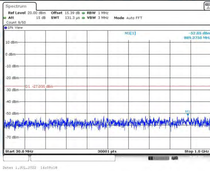
11AX20MIMO_Ant2_5300_30~1000
