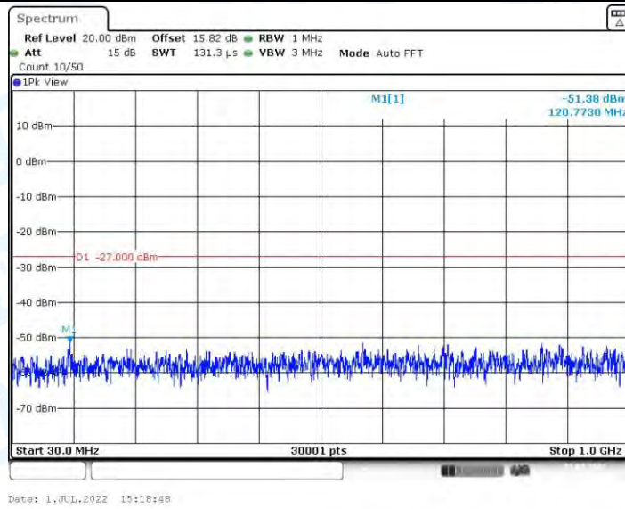
11AX40MIMO_Ant1_5710_30~1000
