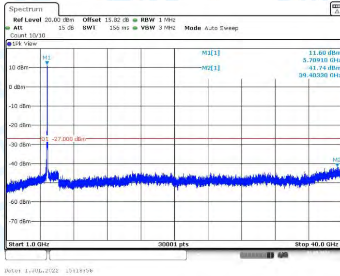
11AX40MIMO_Ant1_5710_1000~40000
