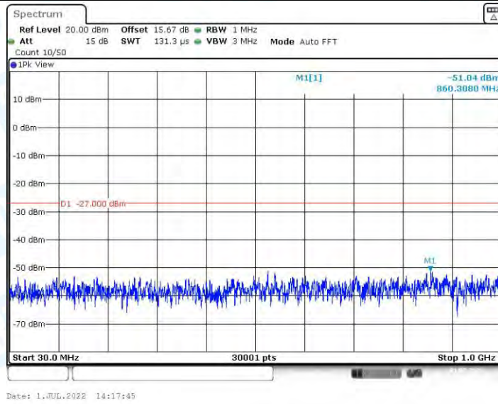
11AX20MIMO_Ant2_5500_30~1000
