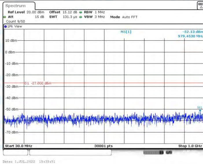
11AX80MIMO_Ant2_5210_30~1000
