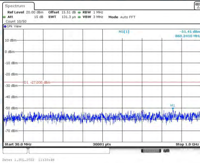
11AC40MIMO_Ant1_5550_30~1000
