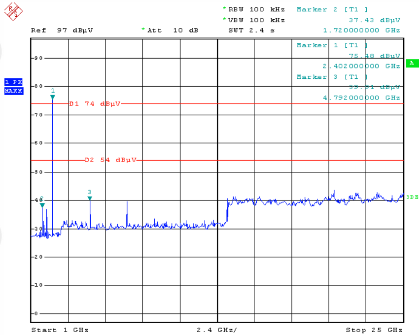
2402MHz (1GHz~25GHz)
