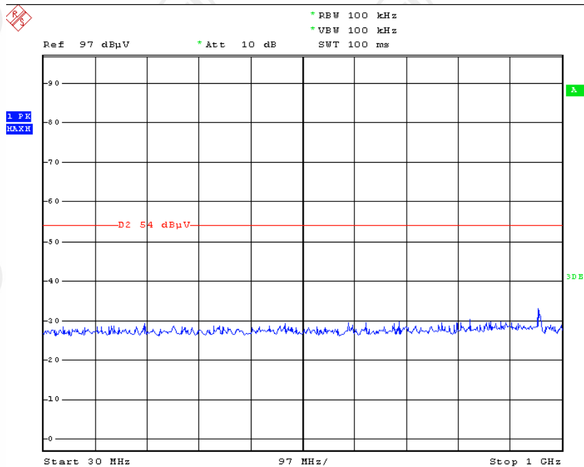
2440MHz (30MHz~1GHz)
