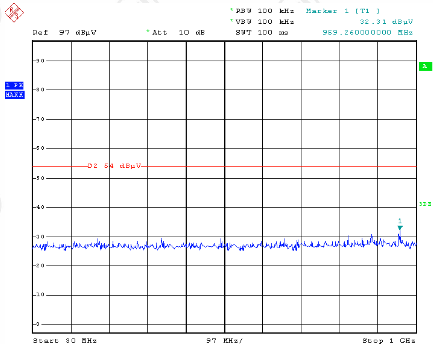
2480MHz (30MHz~1GHz)
