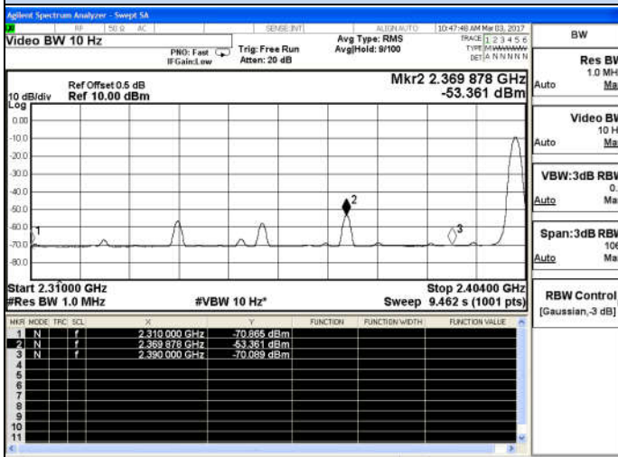
Channel 0 / 2402 MHz – Non-Hopping – AV
