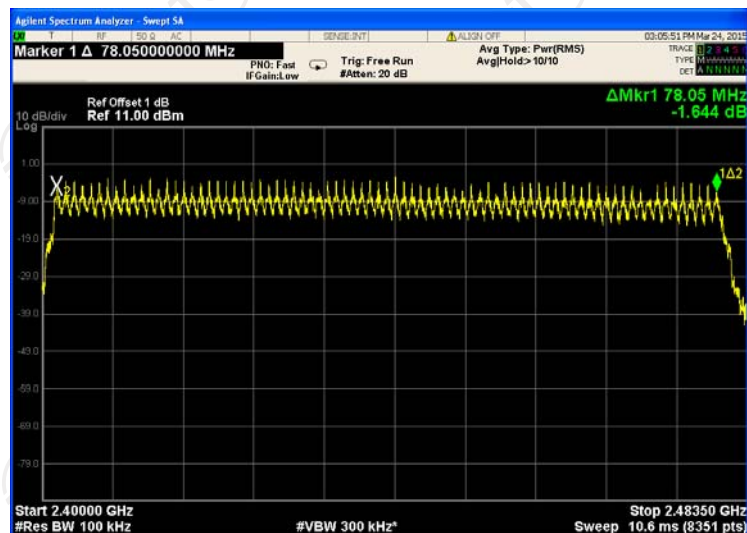
Pi/4DQPSK
