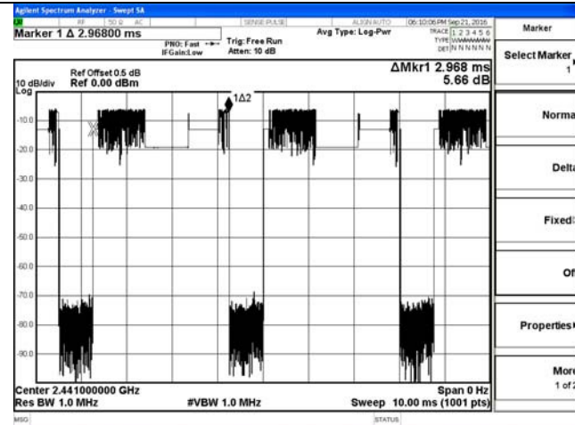
3DH5-2441MHz)
