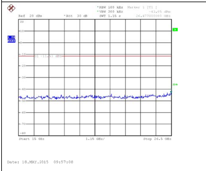
15GHz~26.5GHz
