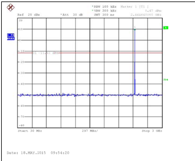
30MHz~3GHz
