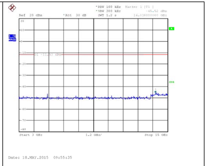
3GHz~15GHz
