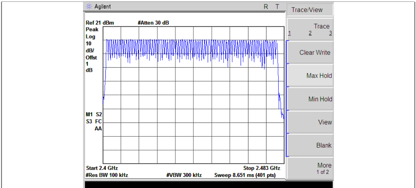
GFSK
