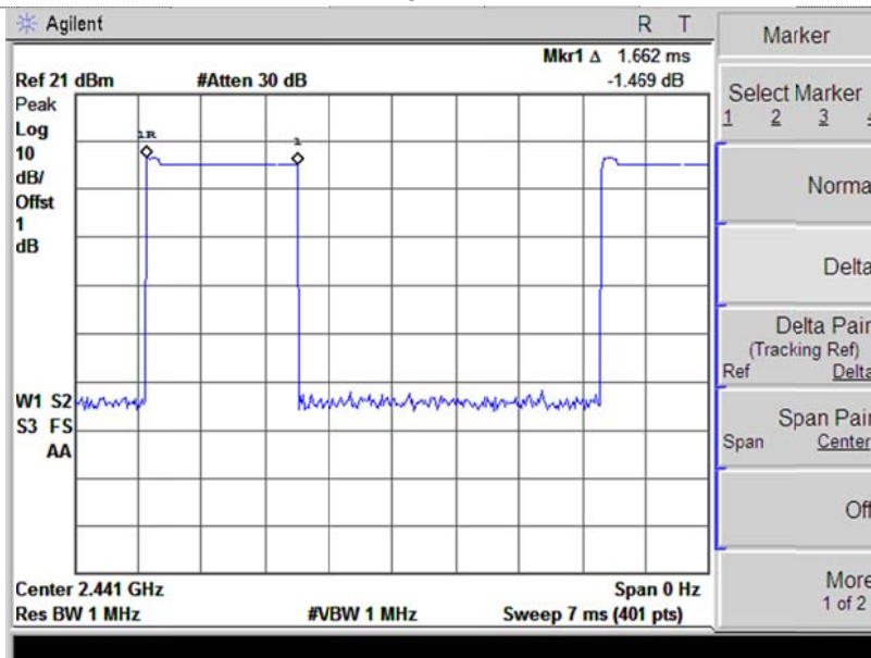
3-DH2
