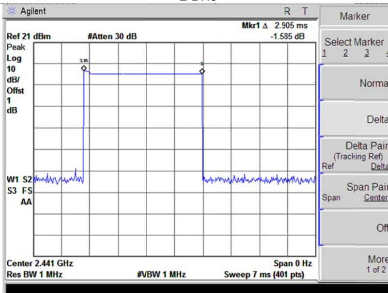
2-DH5
