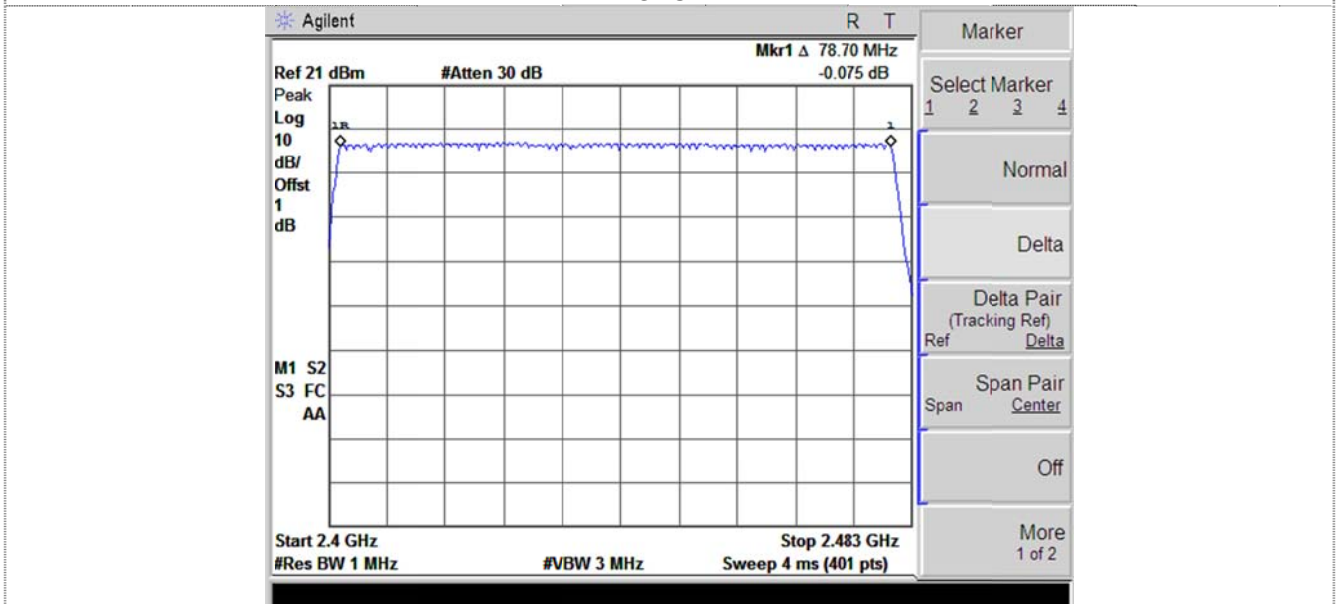
\pi/4 DQPSK
