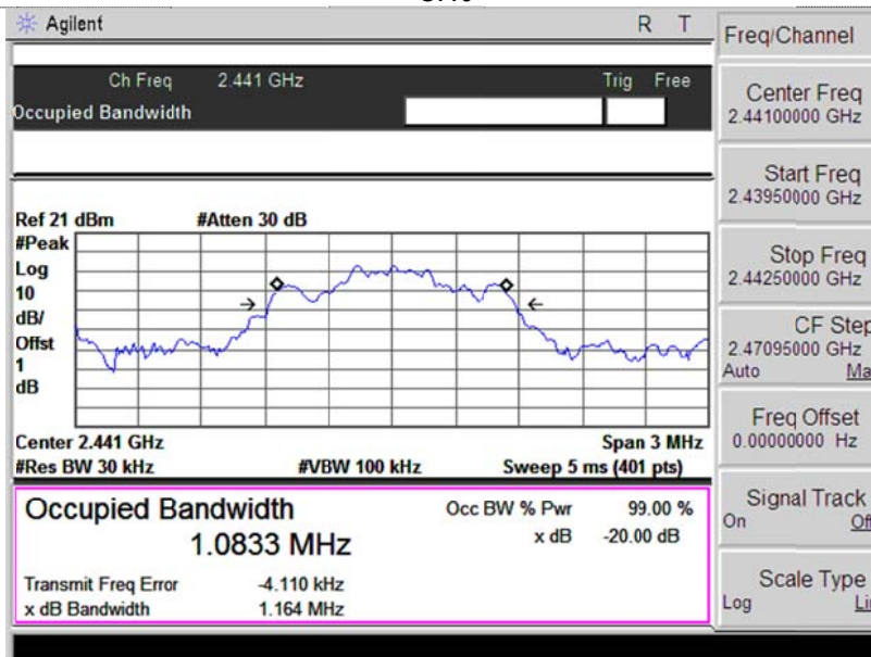
CH39
