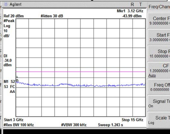
3GHz~15GHz
