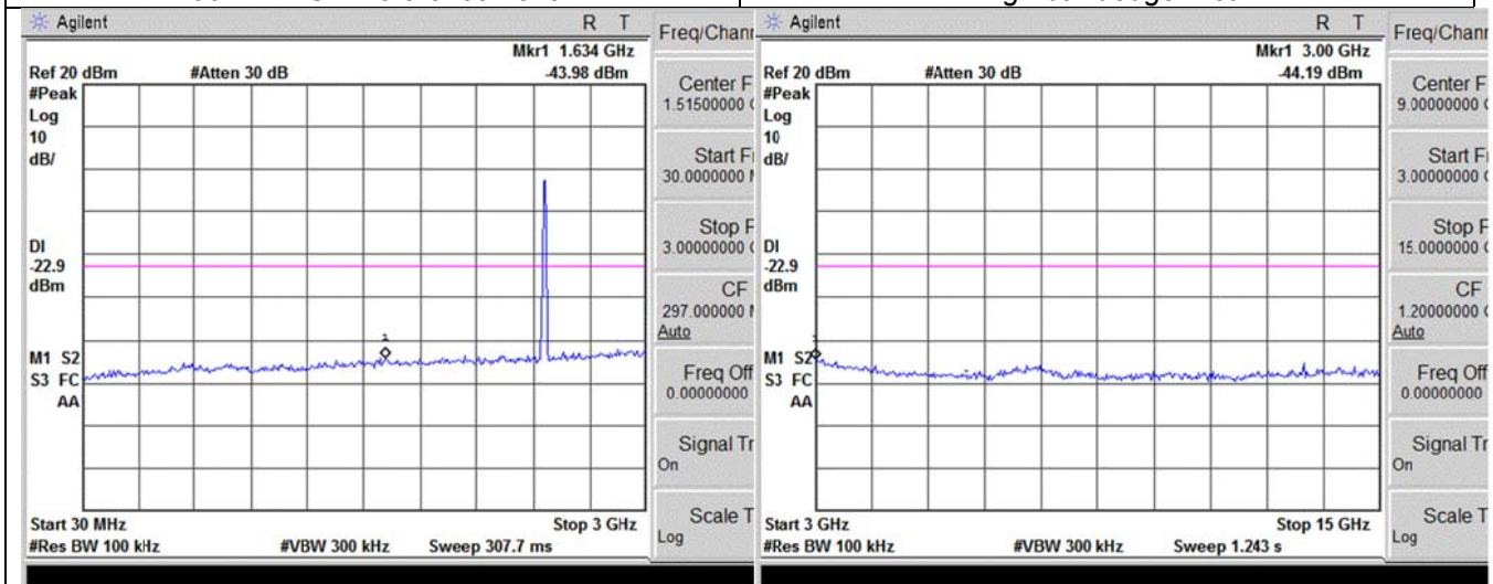
30MHz~3GHz
