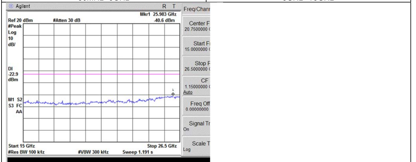
15GHz~26.5GHz
