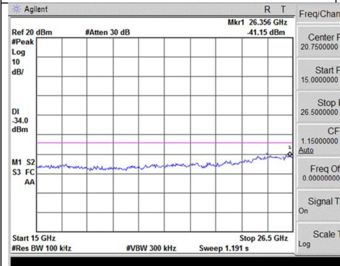
15GHz~26.5GHz
