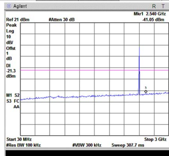
30MHz~3GHz
