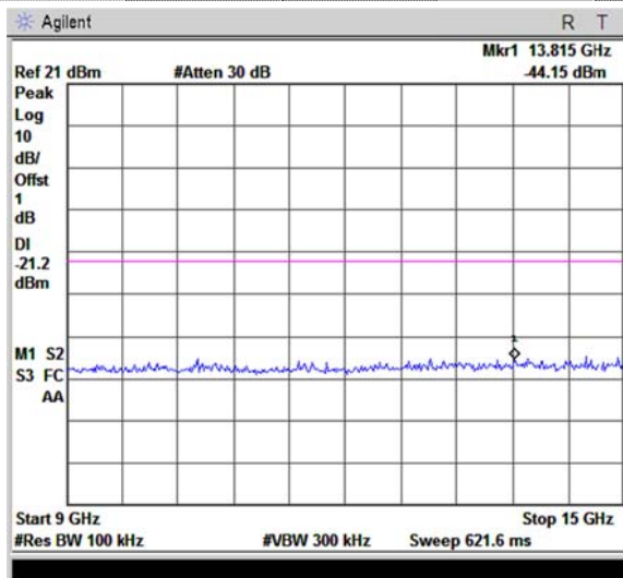
9GHz~15GHz
