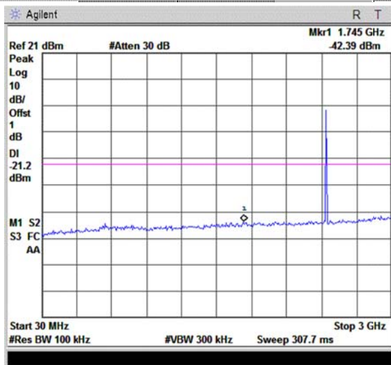
30MHz~3GHz
