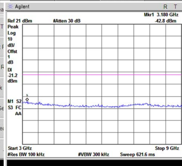
3GHz~9GHz
