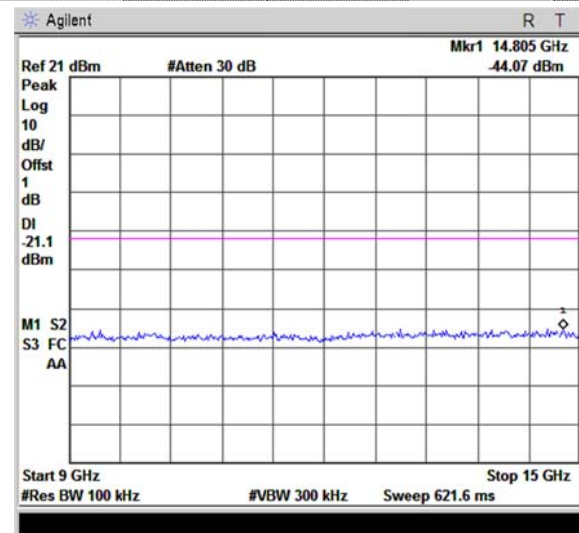
9GHz~15GHz
