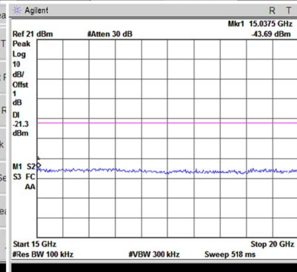
15GHz~20GHz
