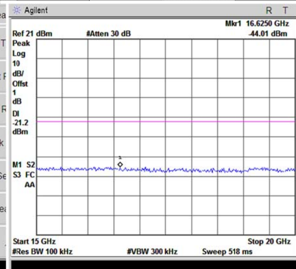
15GHz~20GHz
