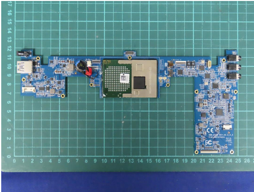
(12) EUT Photo
