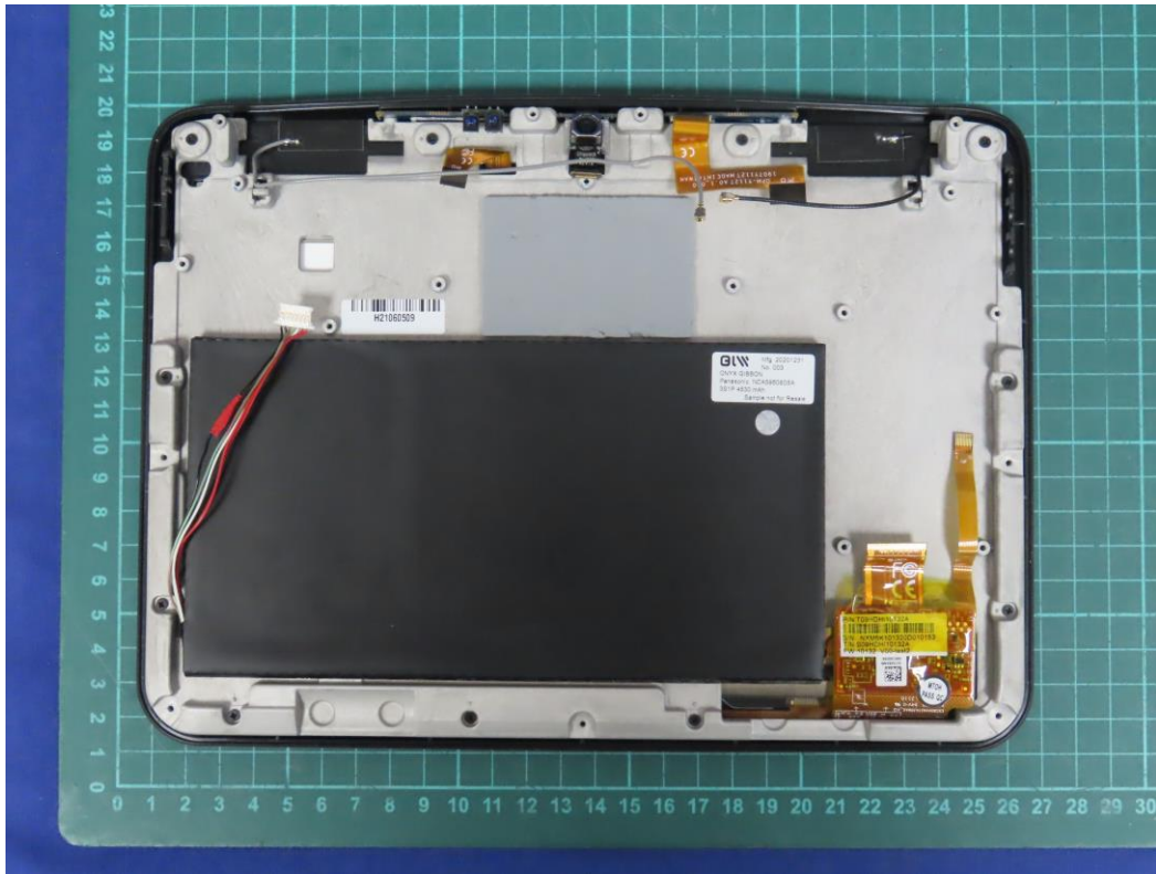
(20) EUT Photo
