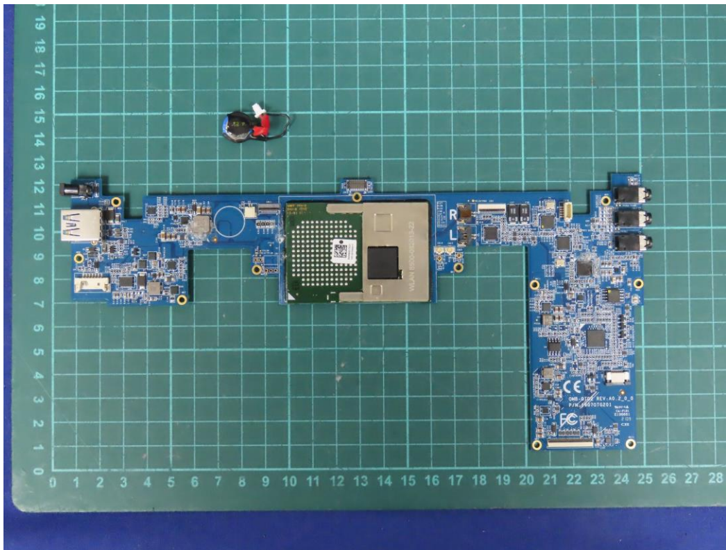
(13) EUT Photo
