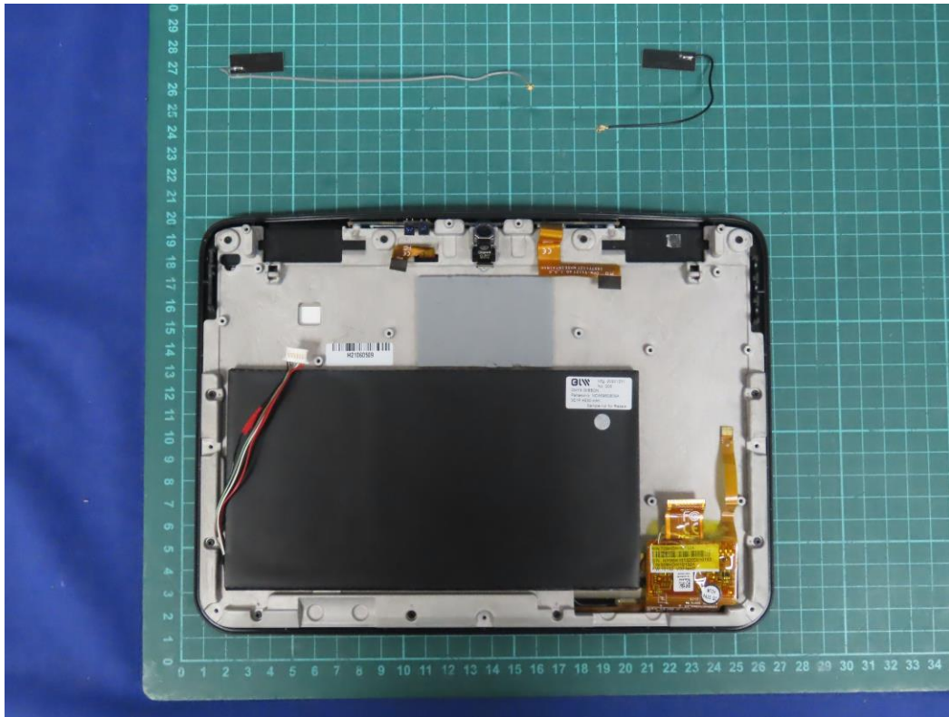
(21) EUT Photo
