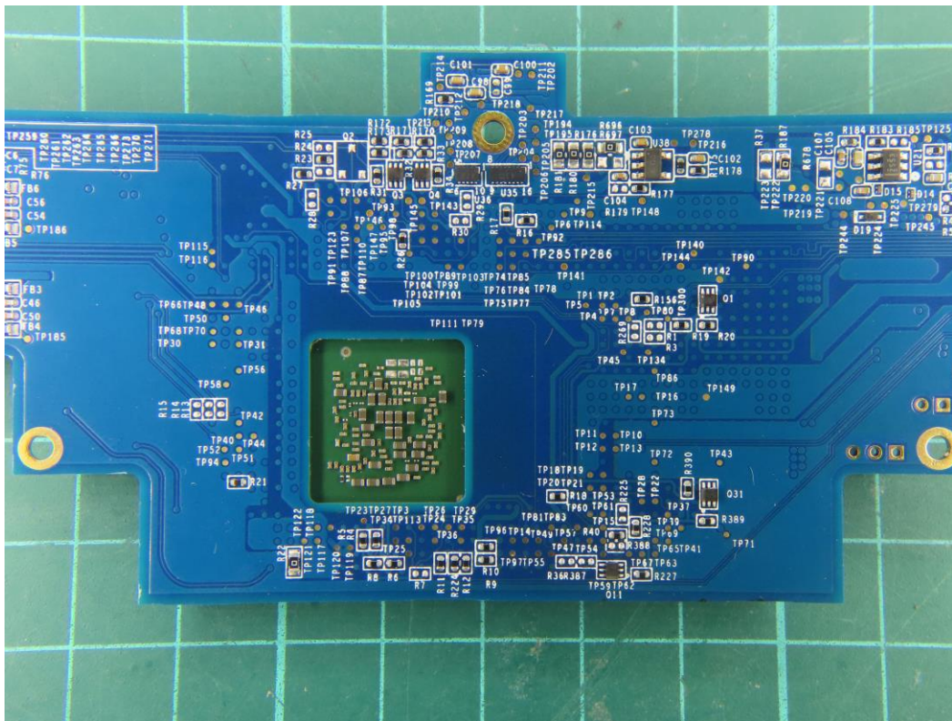
(19) EUT Photo
