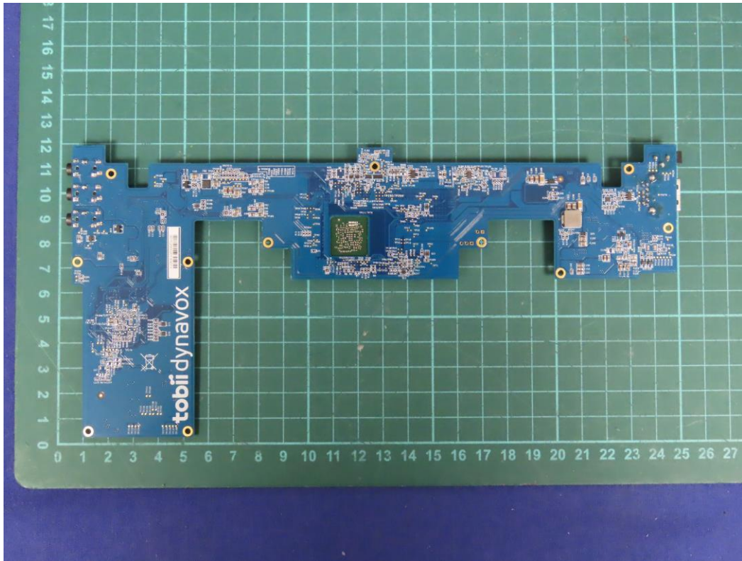
(18) EUT Photo
