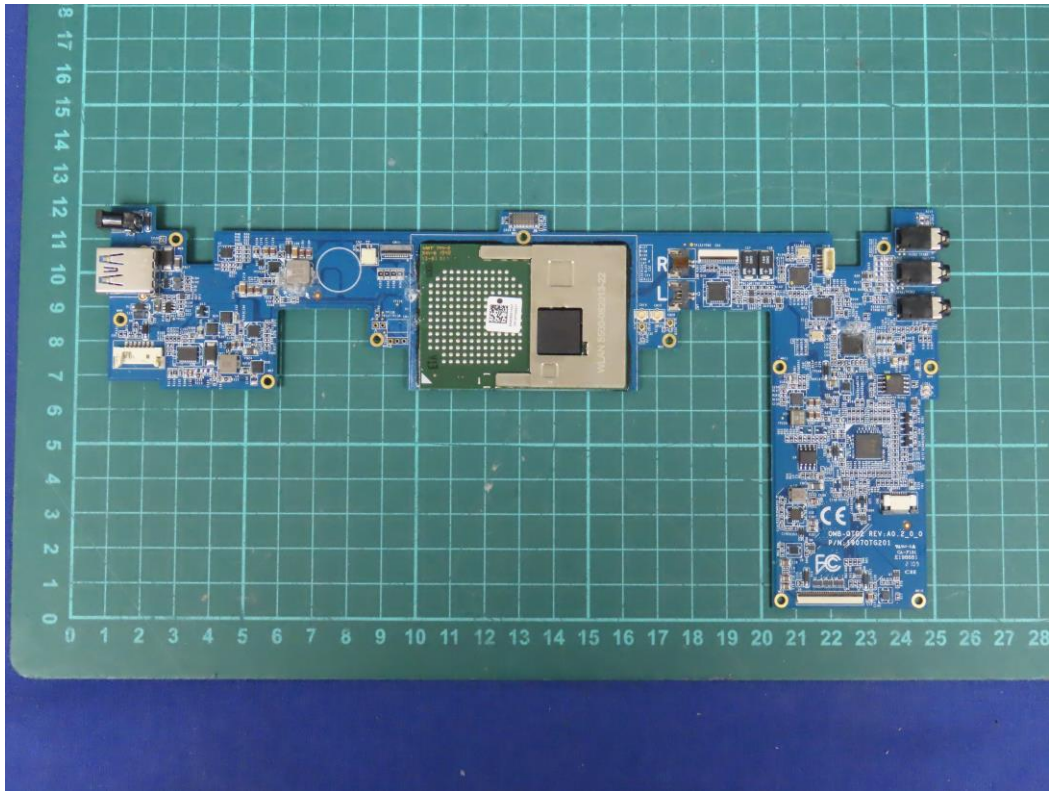
(14) EUT Photo
