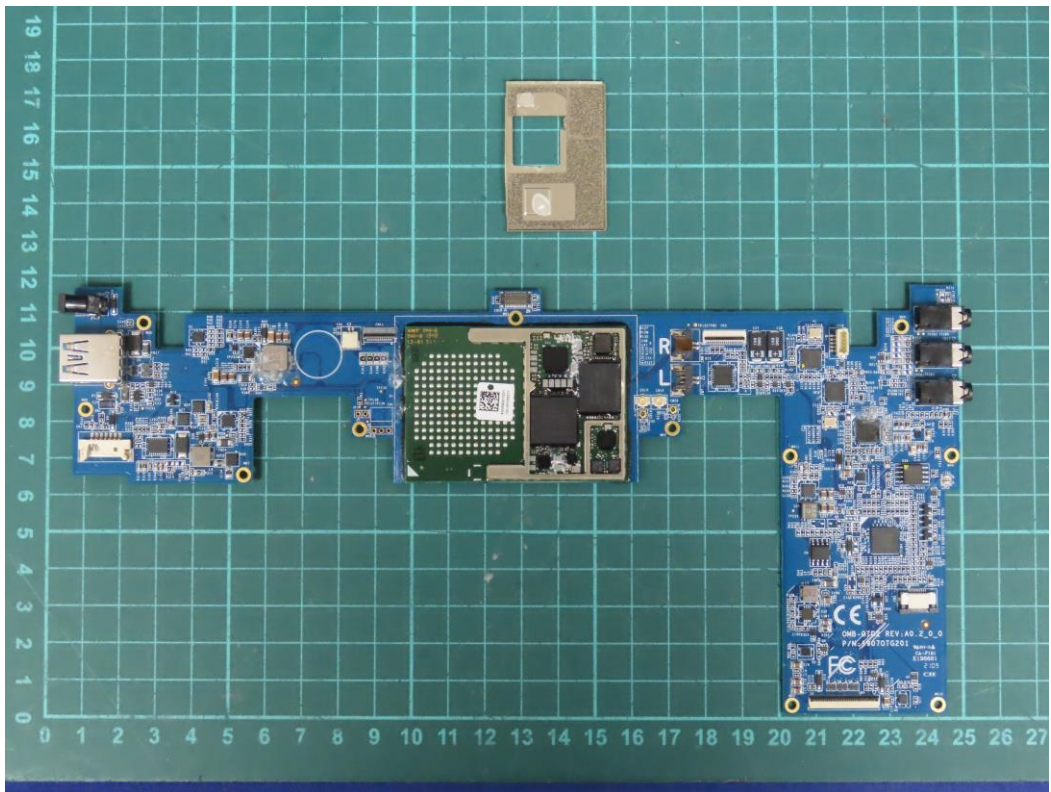
(15) EUT Photo
