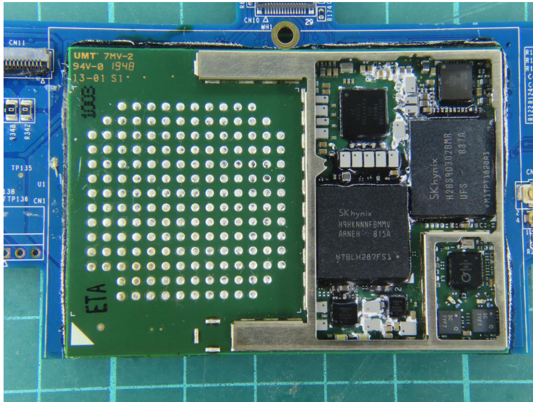
(16) EUT Photo
