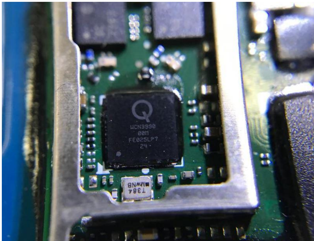
(17) EUT Photo
