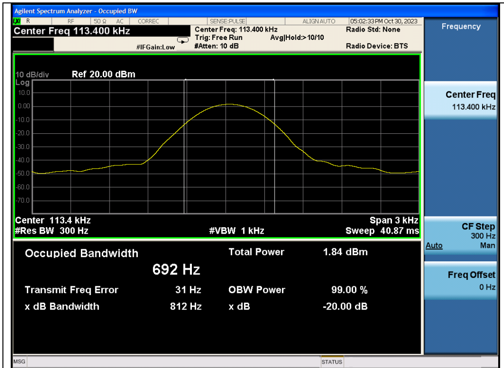
Test_Graph_ASK_Coil ANT_ 113.4kHz _ -20dB Bandwidth
