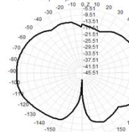
2420.0MHz Total(E2-YZ), Max: -7.53dBi
