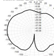
2410.0MHz Total(E2-YZ), Max: -7.32dBi
