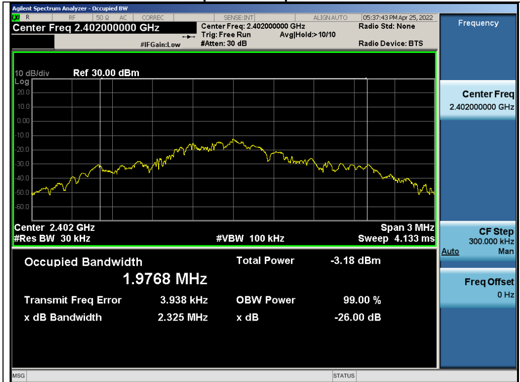
Test_Graph_2.4GHz_ANT1_2402_GFSK_OBW
