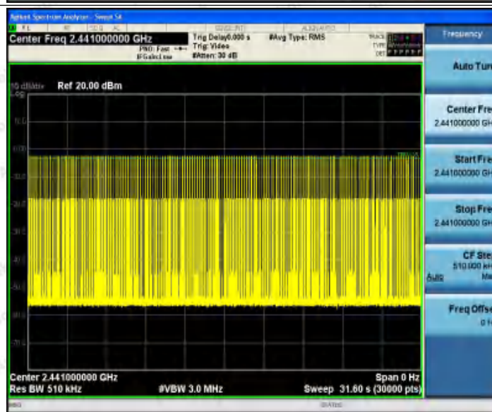
2DH3_Ant1_Hop
