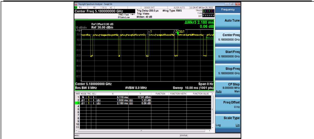
11AC20MIMO_Ant2_5180
