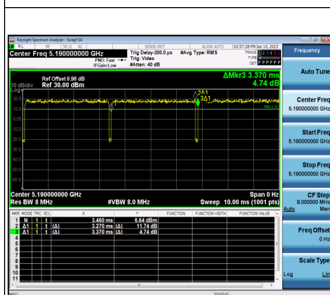
802.11n HT40
