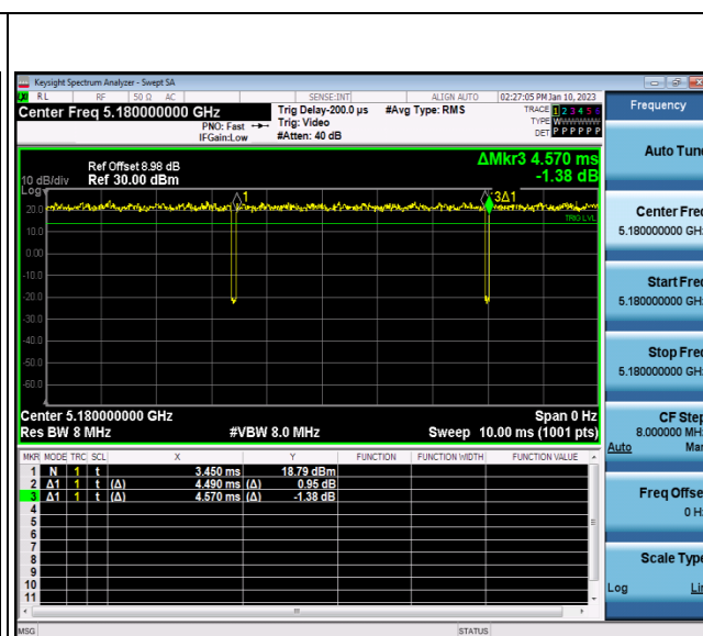
802.11n HT20
