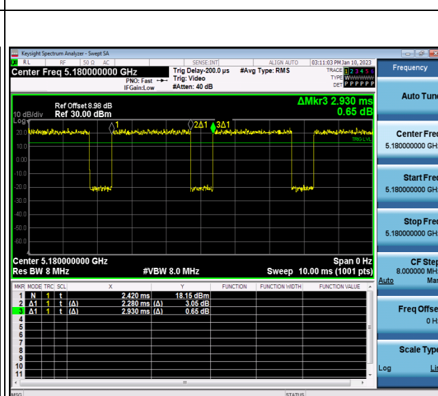
802.11ac VHT20
