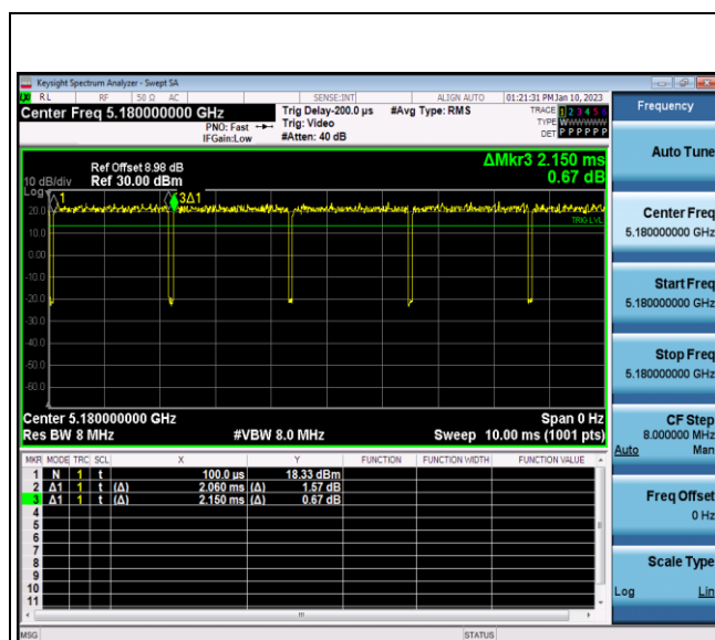
802.11a
