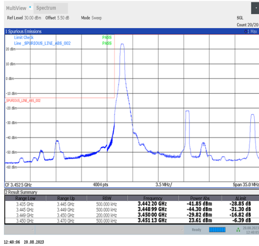
Band42_20MHz_QPSK_42190_1RB#0
