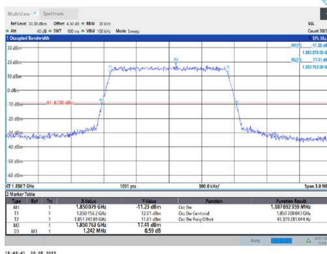
Band25-1.4MHz-QPSK-26365-6RB#0
