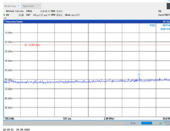
Band25-20MHz-QPSK-26140-1RB#0-Range2:0.15~30MHz
