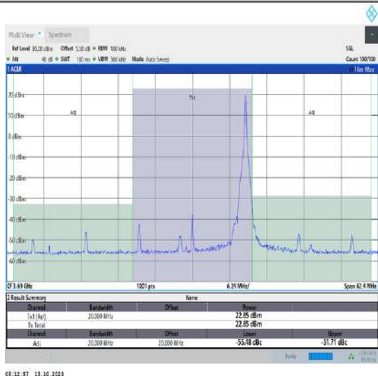
43(3600-3700)-20MHz-QPSK-44490-1RB#99-PASS
