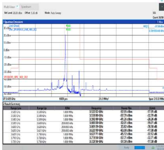
Band43_20MHz_QPSK_43690_1RB#0
