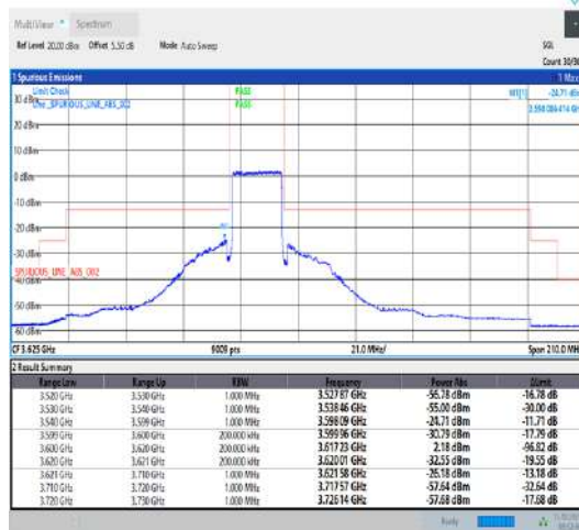
Band43_20MHz_QPSK_43690_100RB#0
