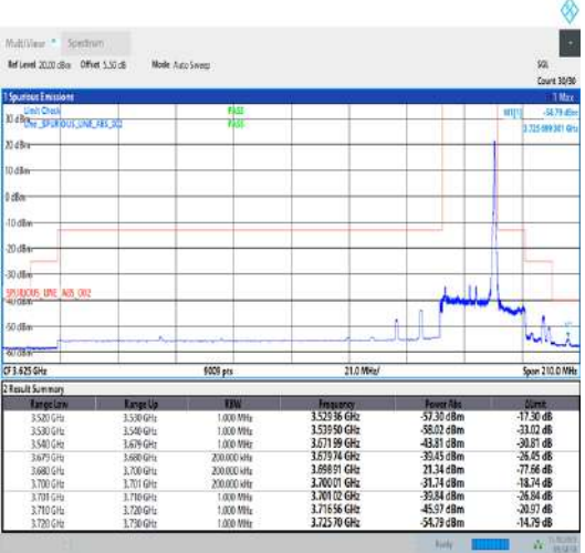
Band43_20MHz_QPSK_44490_1RB#99
