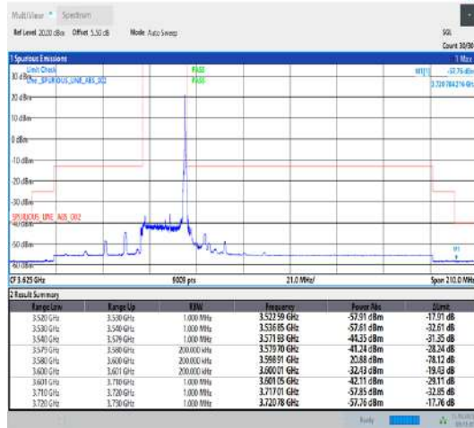
Band42_20MHz_QPSK_43490_1RB#99
