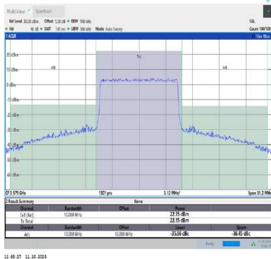
42(3550-3600)-10MHz-QPSK-43340-50RB#0-PASS
