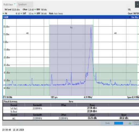
42(3550-3600)-20MHz-QPSK-43190-1RB#99-PASS
