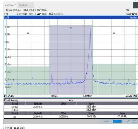
42(3550-3600)-20MHz-QPSK-43340-1RB#99-PASS
