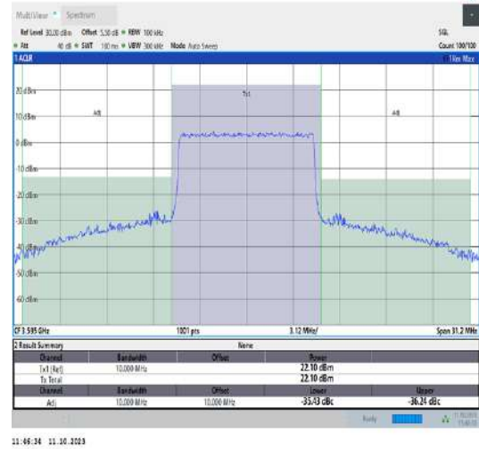
42(3550-3600)-10MHz-QPSK-43540-50RB#0-PASS
