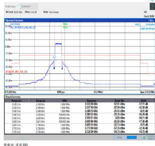
Band42_10MHz_QPSK_43540_50RB#0
