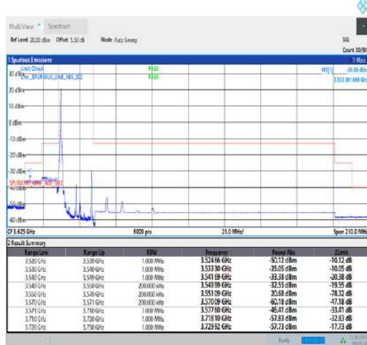
Band42_20MHz_QPSK_43490_1RB#99
