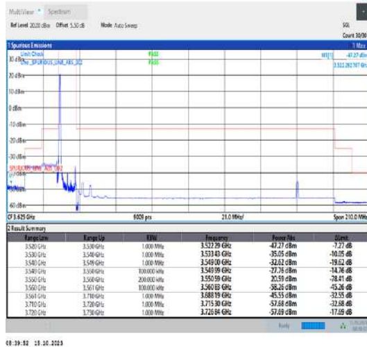
Band42_10MHz_QPSK_43140_1RB#0
