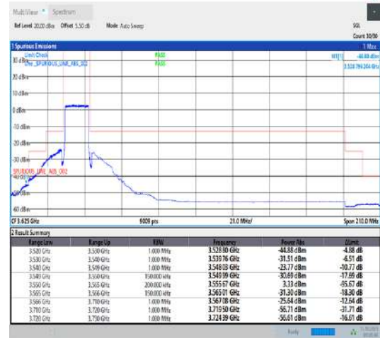
Band42_15MHz_QPSK_43165_75RB#0
