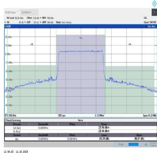
42(3550-3600)-10MHz-QPSK-43140-50RB#0-PASS
