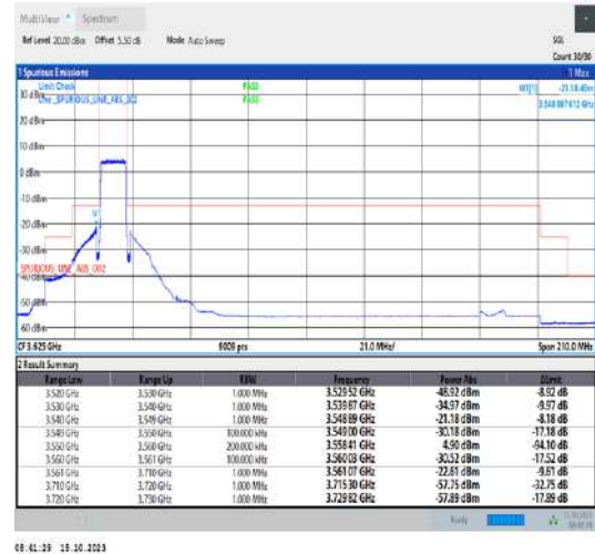
Band42_10MHz_QPSK_43140_50RB#0
