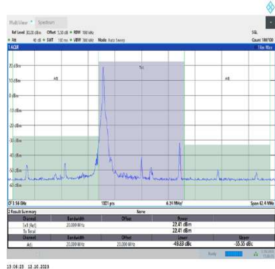
42(3550-3600)-20MHz-QPSK-43190-1RB#0-PASS
