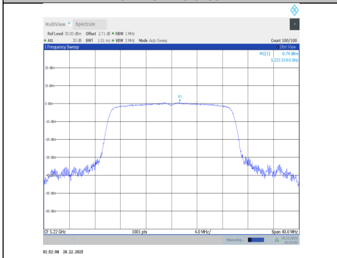
11ax20MIMO-Ant1-5220-PASS
