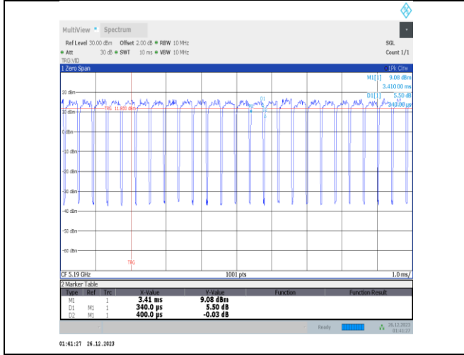
NTNV-11ax40MIMO-Ant1-5190
