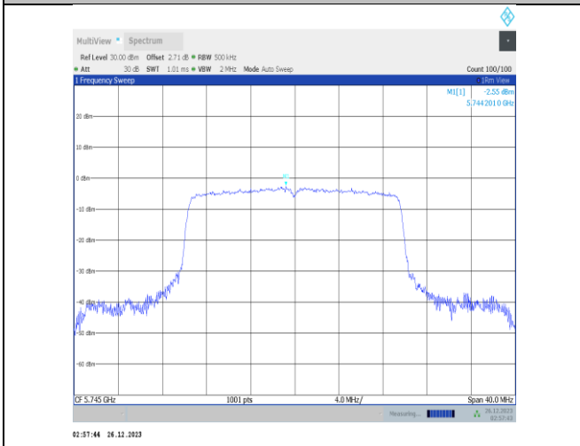
11x20MIMO-Ant1-5745-PASS
