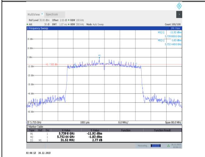
11ax40MIMO-Ant3-5755-PASS
