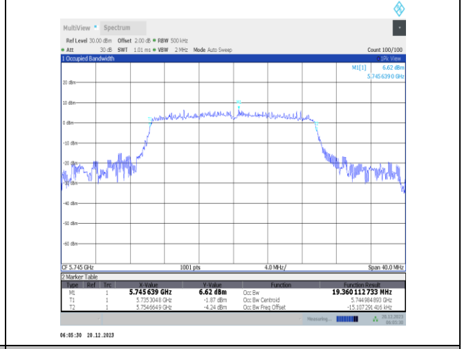
11ax20MIMO-Ant2-5745
