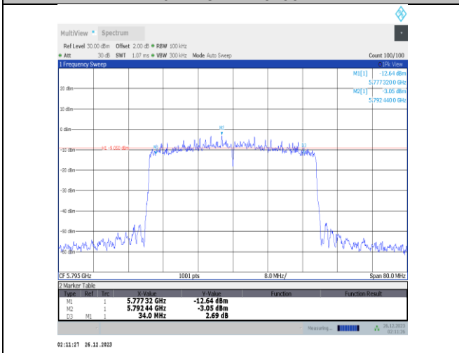
11ax40MIMO-Ant3-5795-PASS
