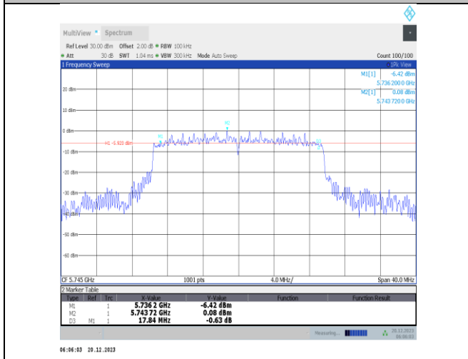
11ax20MIMO-Ant3-5745-PASS
