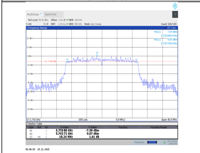
11ax20MIMO-Ant1-5745-PASS
