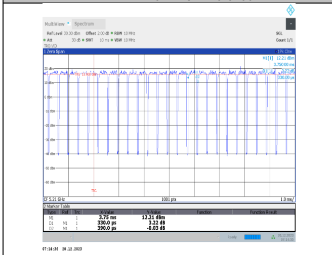
NTNV-11ac80MIMO-Ant1-5210
