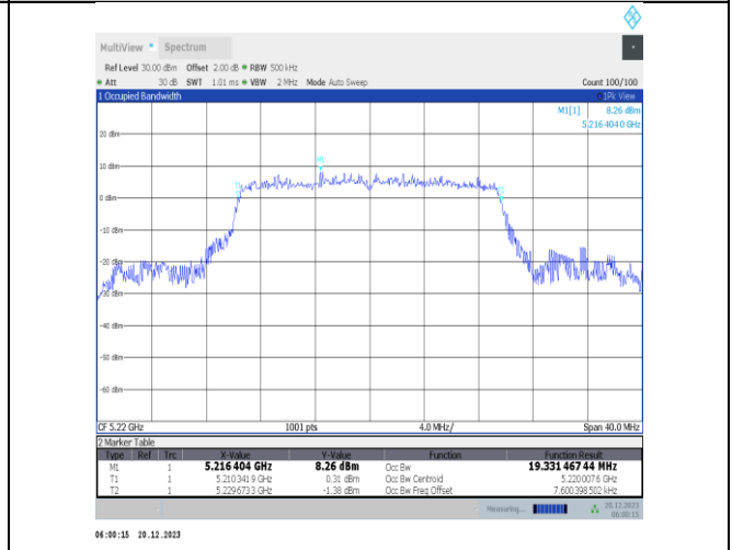
11ax20MIMO-Ant2-5220
