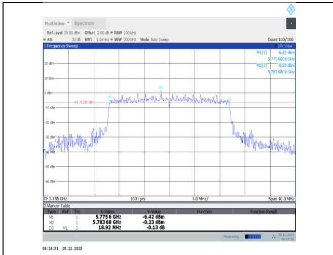
11ax20MIMO-Ant1-5785-PASS
