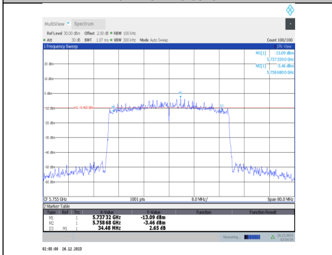
11ax40MIMO-Ant1-5755-PASS
