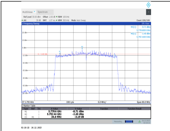
11ax40MIMO-Ant1-5795-PASS
