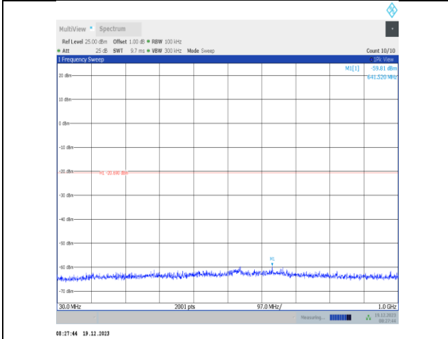
11ax20MIMO-Ant3-2437-30~1000-PASS
