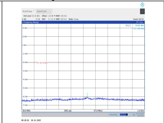
11ax20MIMO-Ant4-2437-30~1000-PASS
