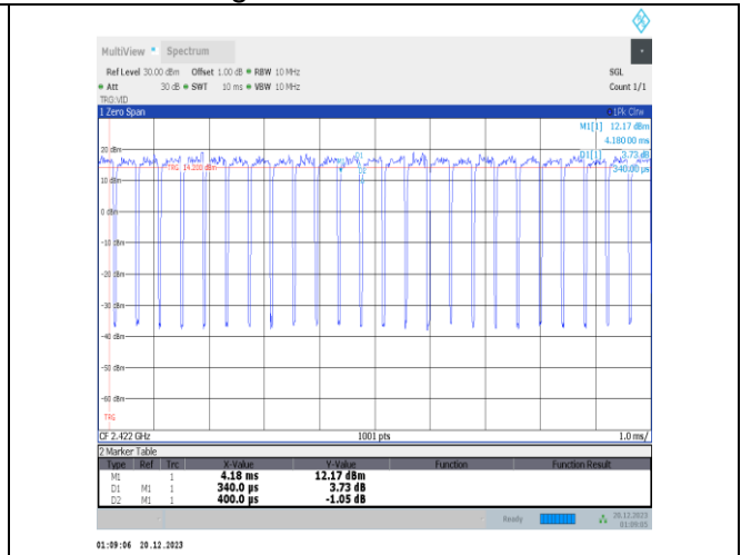
NTNV-11ax40MIMO-Ant3-2422
