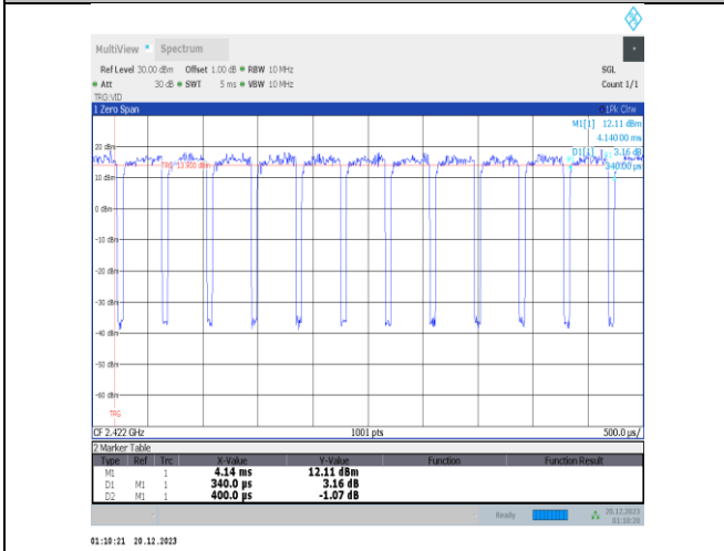
NTNV-11ax40MIMO-Ant4-2422
