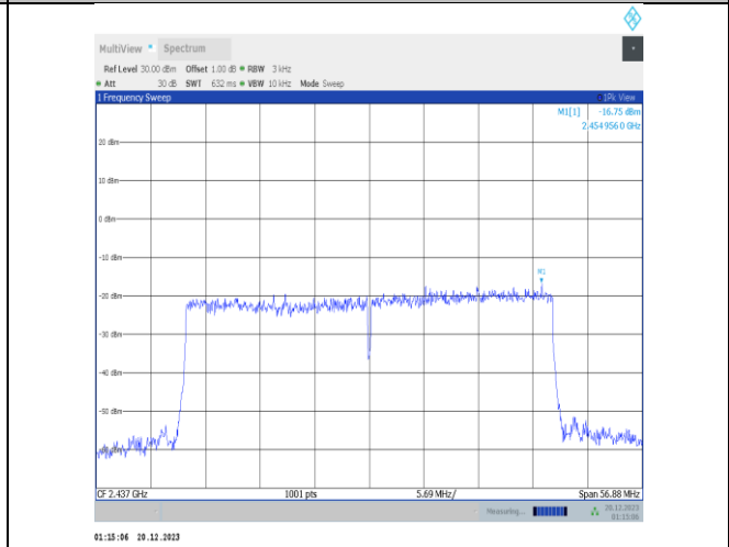
11ax40MIMO-Ant3-2437-PASS
