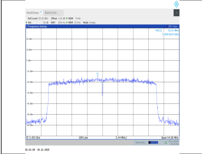
11ax40MIMO-Ant4-2452-PASS
