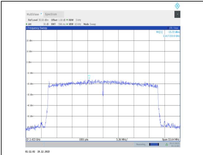
11ax40MIMO-Ant4-2422-PASS
