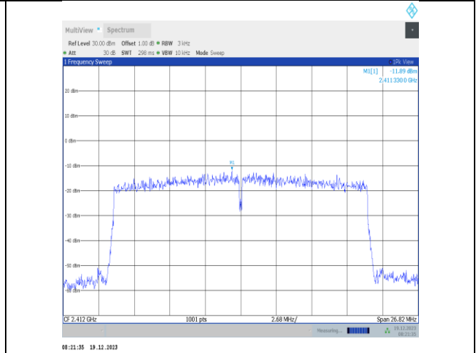
11ax20MIMO-Ant3-2412-PASS
