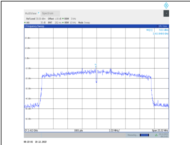
11ax20MIMO-Ant4-2412-PASS
