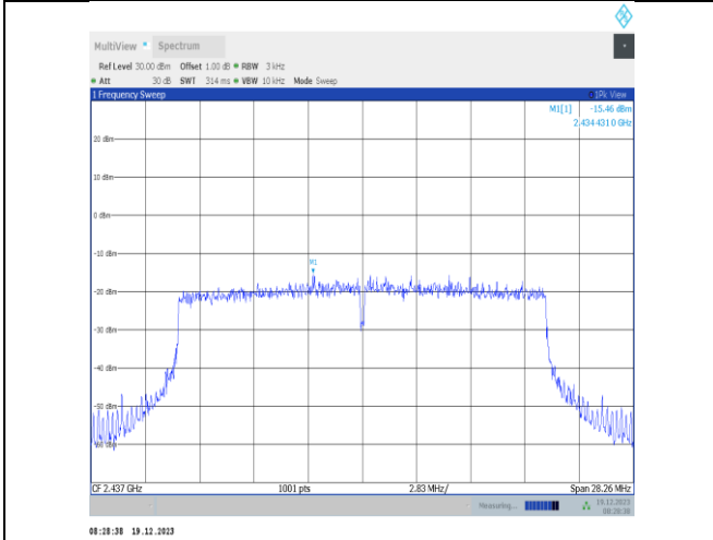
11ax20MIMO-Ant4-2437-PASS
