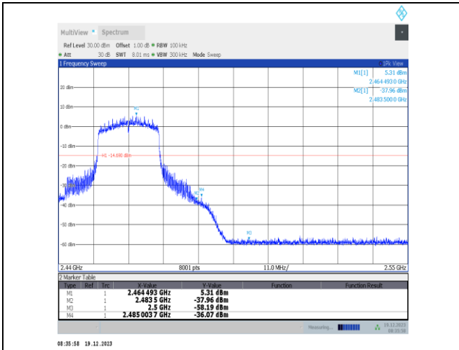
11ax20MIMO-Ant4-2462-PASS
