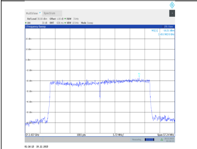
11ax40MIMO-Ant4-2437-PASS
