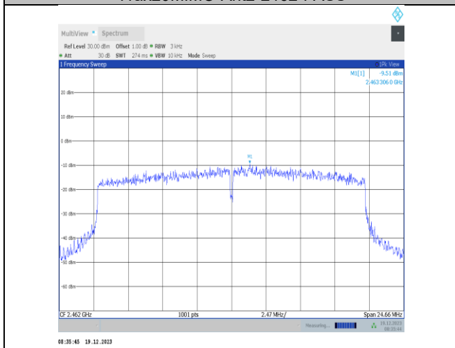
11ax20MIMO-Ant4-2462-PASS
