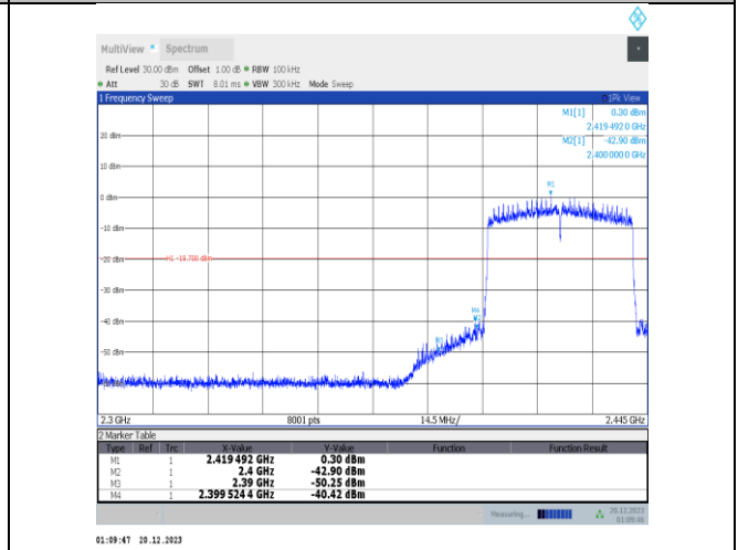
11ax40MIMO-Ant3-2422-PASS
