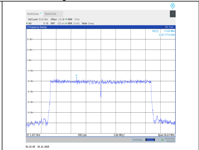
11ax40MIMO-Ant1-2437-PASS
