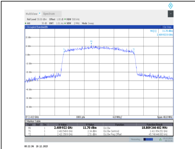
11ax20MIMO-Ant4-2412
