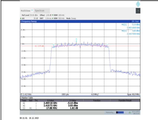
11ax20MIMO-Ant3-2412-PASS
