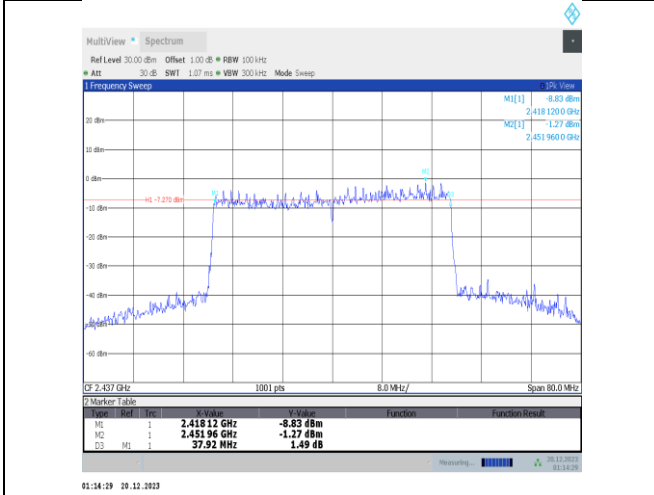
11ax40MIMO-Ant3-2437-PASS
