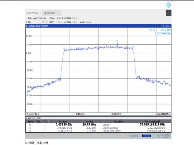
11ax40MIMO-Ant3-2422
