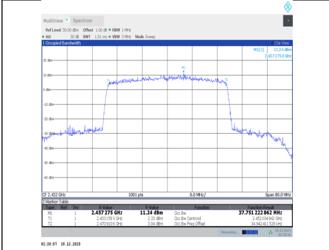
11x40MIMO-Ant4-2452
