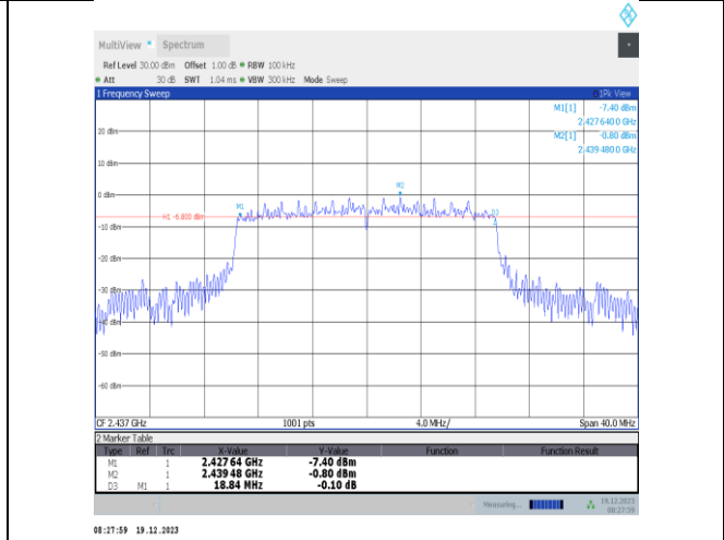
11x20MIMO-Ant4-2437-PASS
