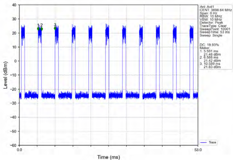
n48_30kHz_SISO_NTNV_20MHz_CP-OFDM_256_QAM_3690MHz_Inner_1RB_Right_Ant1
