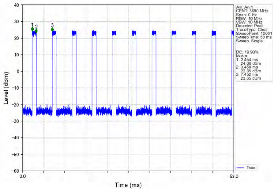
n48_30kHz_SISO_NTNV_20MHz_CP-OFDM QPSK_3690MHz_Inner_Full_Ant1
