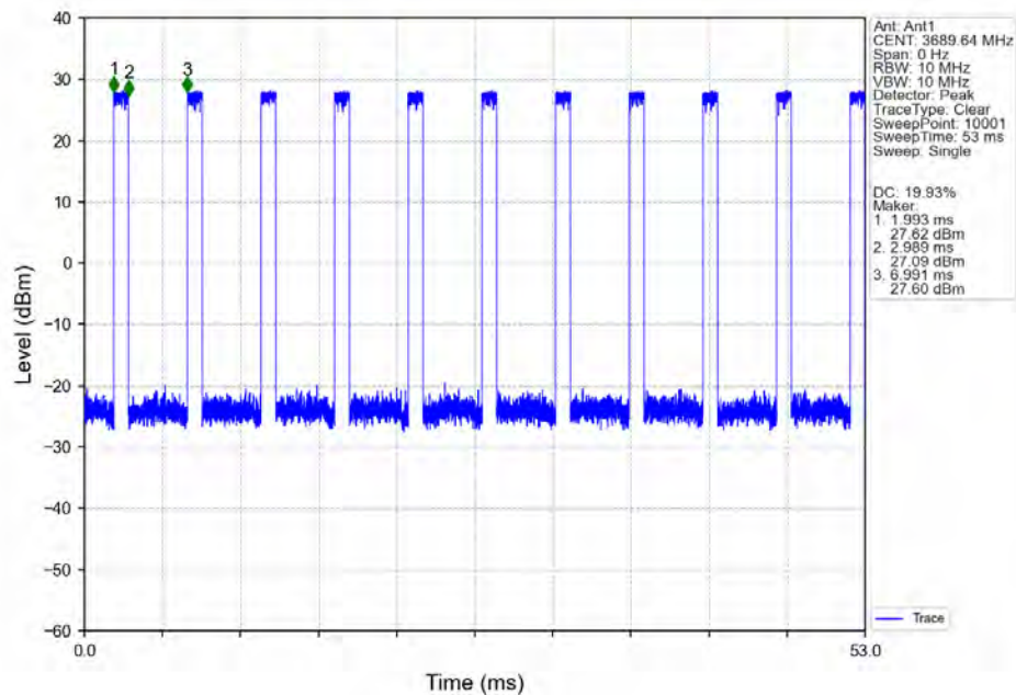
n48_30kHz_SISO_NTNV_20MHz_CP-OFDM_16_QAM_3690MHz_Inner_Full_Ant1
