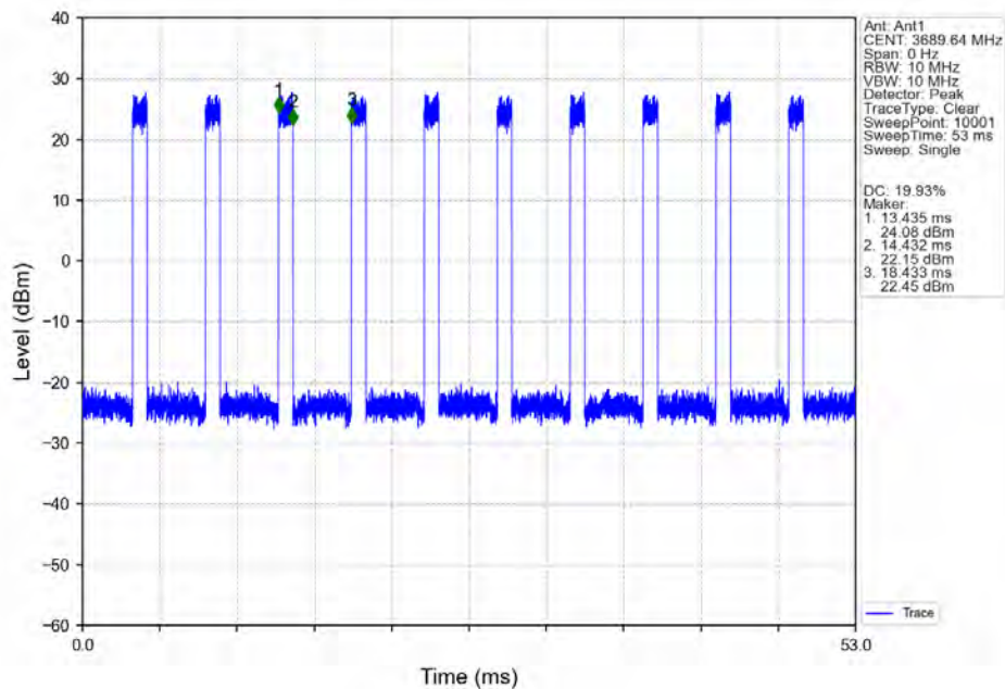
n48_30kHz_SISO_NTNV_20MHz_CP-OFDM_256_QAM_3690MHz_Inner_Full_Ant1
