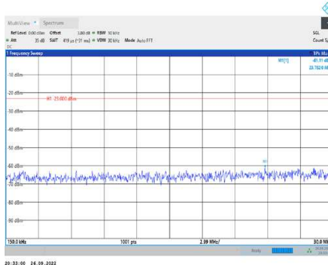
Band71-20MHz-QPSK-133222-1RB#0-Range2:0.15~30MHz
