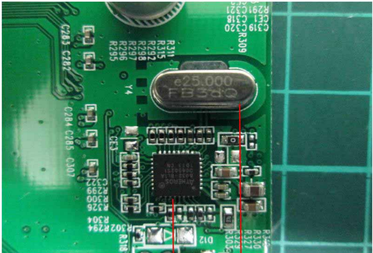
Ethernet phy on VOIP Module
