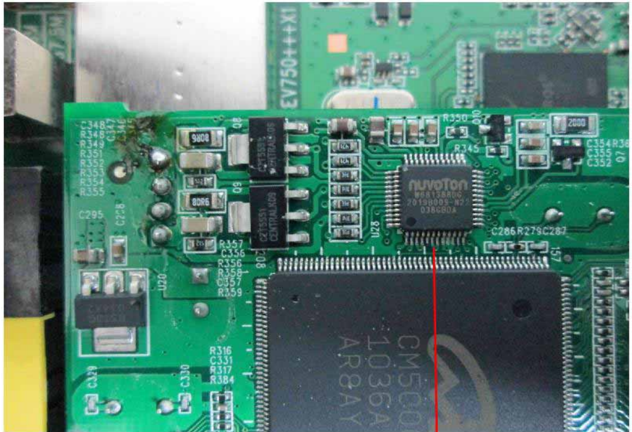
VOIP SLIC
